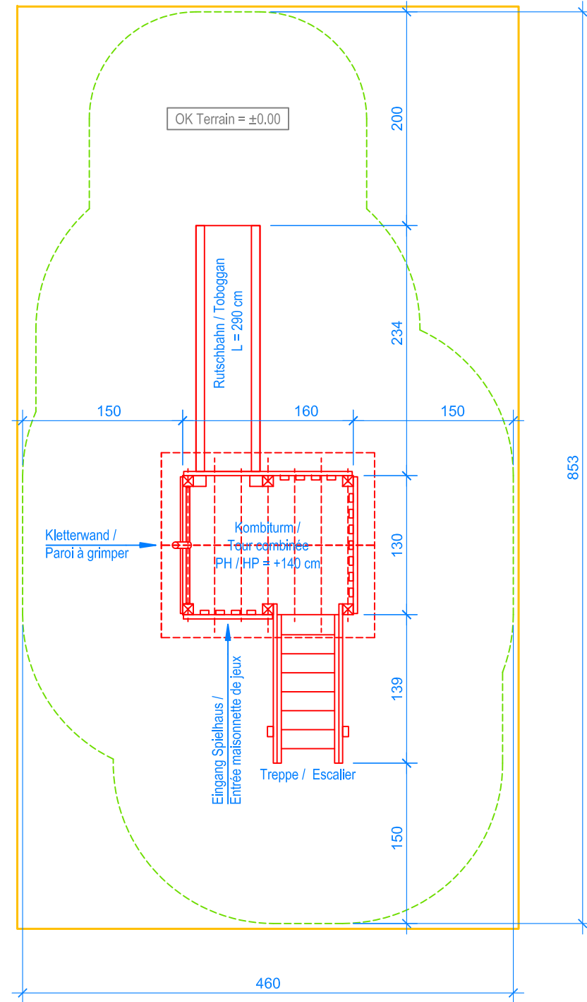
GRUNDRISS / PLAN 1:50
