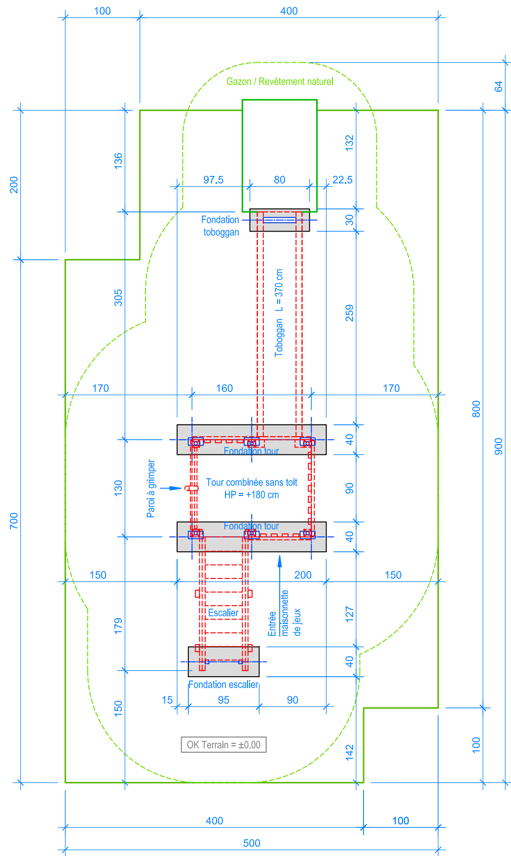
PLAN 1:50
