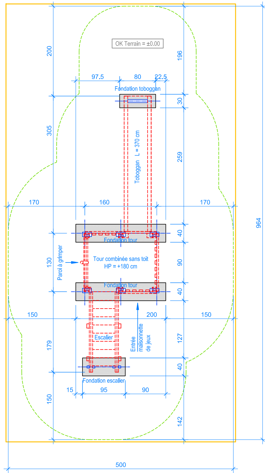
PLAN 1:50
