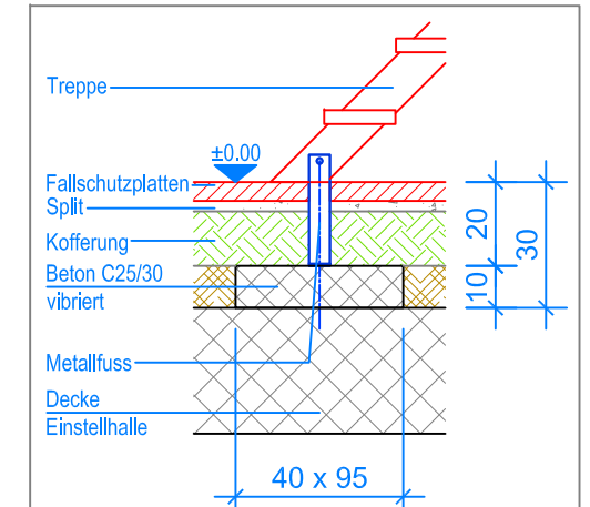
SCHNITT 1:20 FUNDAMENT TREPPE
