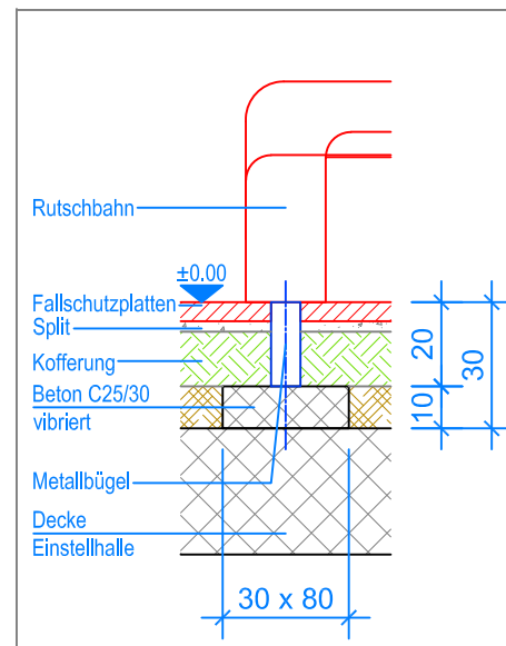
SCHNITT 1:20 FUNDAMENT RUTSCHBAHN
