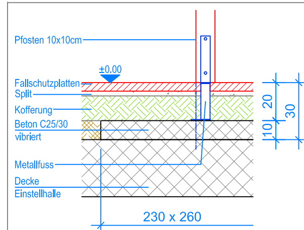
SCHNITT 1:20 FUNDAMENT TURM
