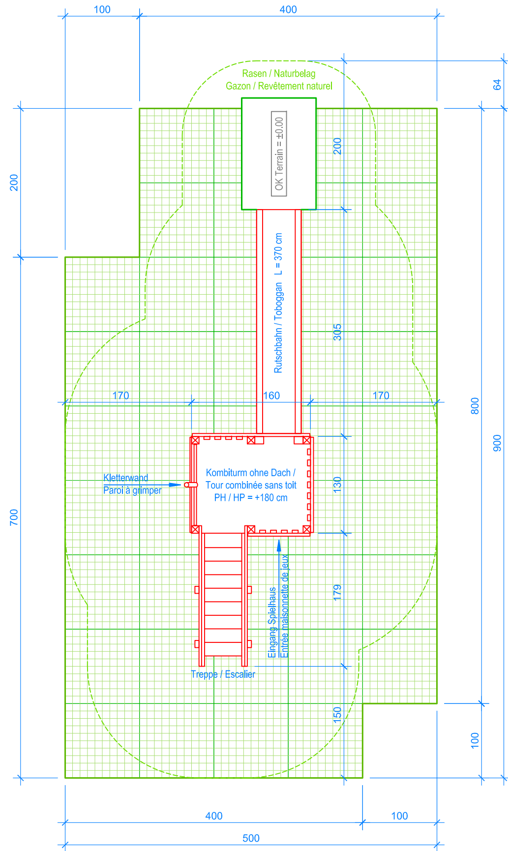
GRUNDRISS / PLAN 1:50
