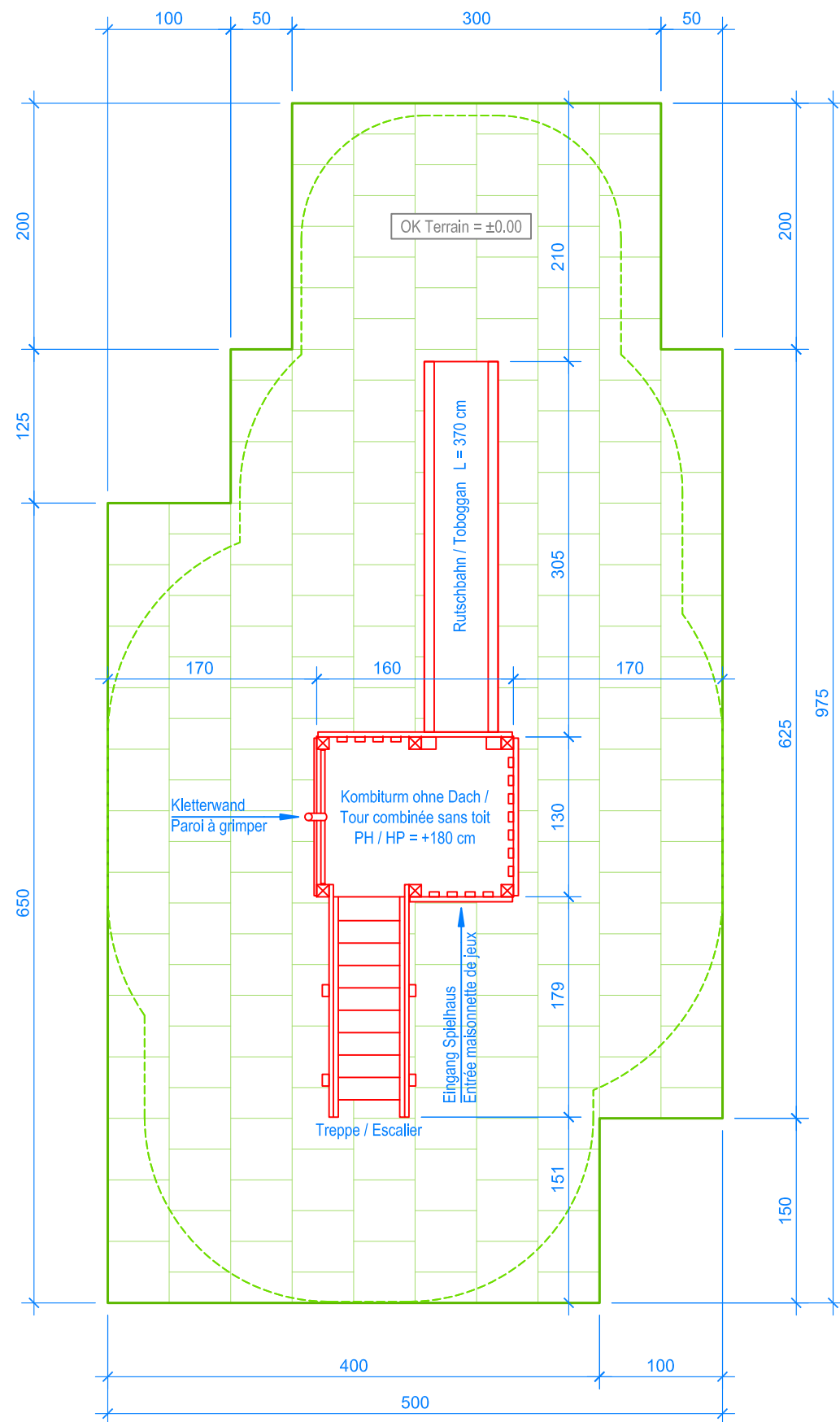
GRUNDRISS / PLAN 1:50
