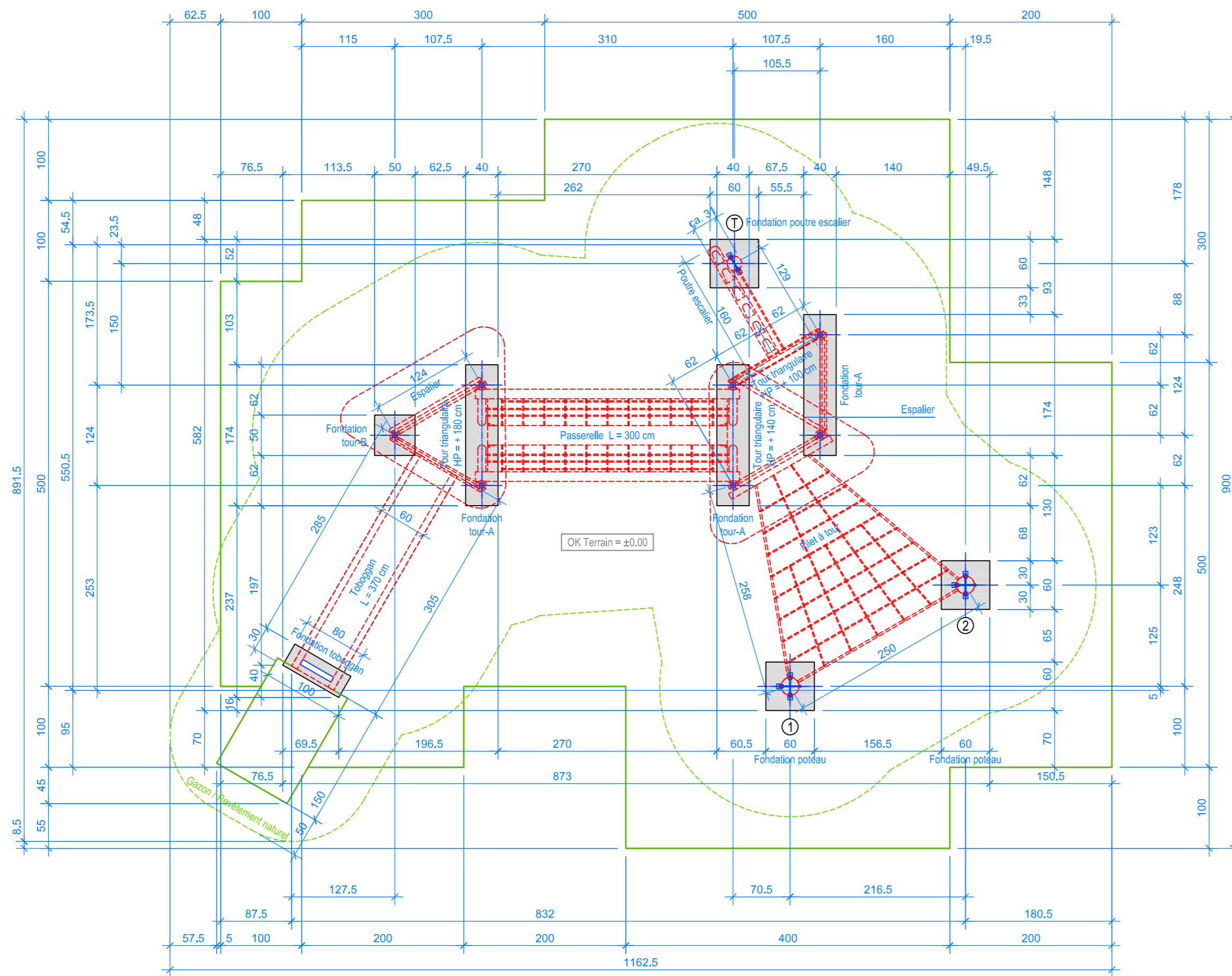
PLAN 1:50
