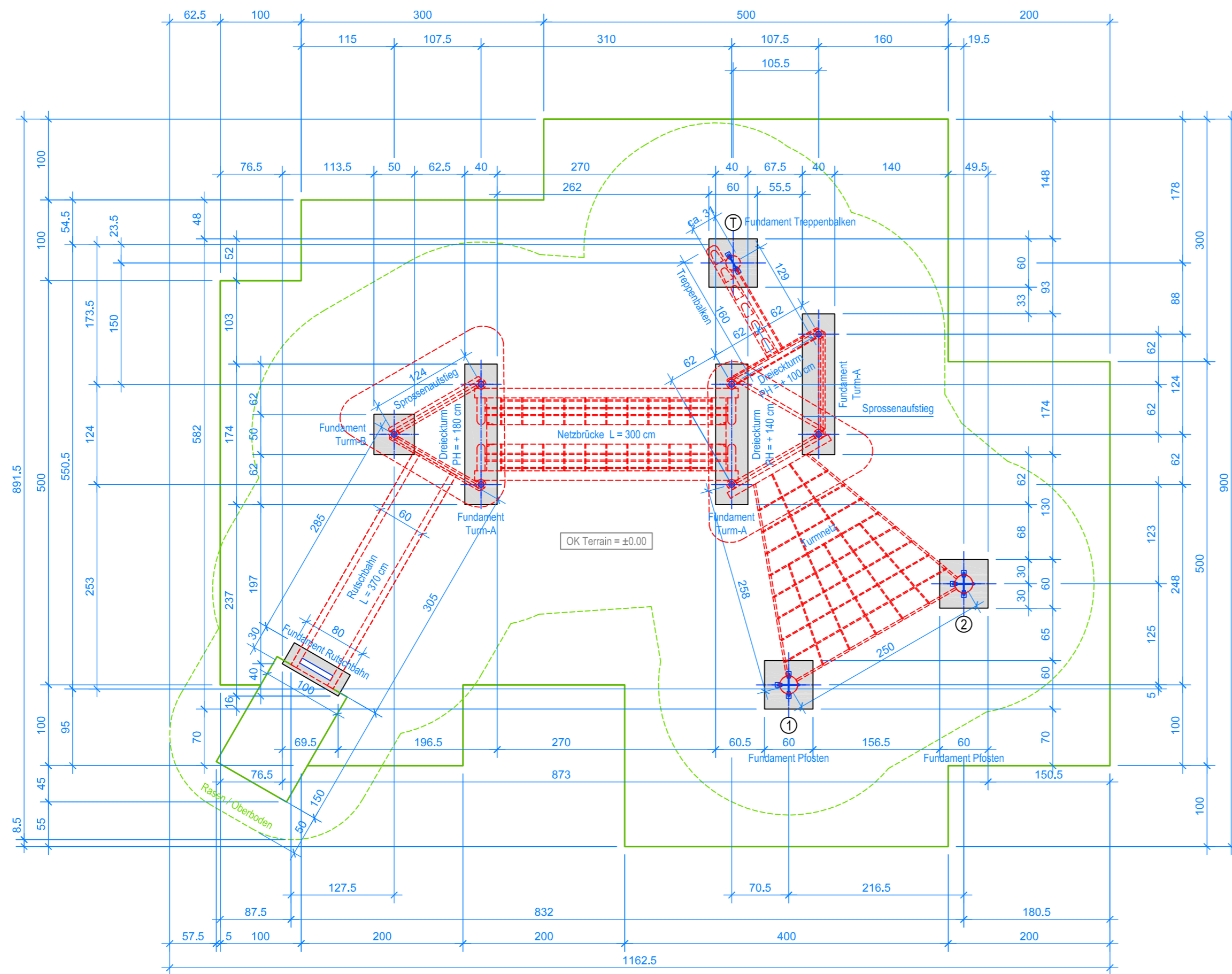
GRUNDRISS 1:50
