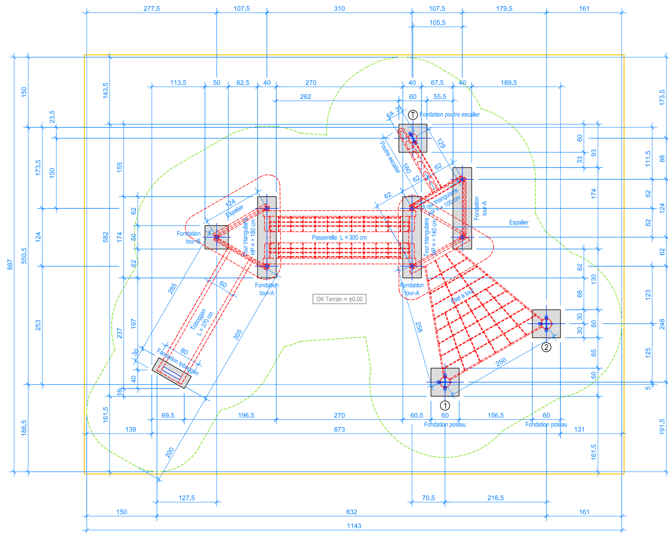
PLAN 1:50
