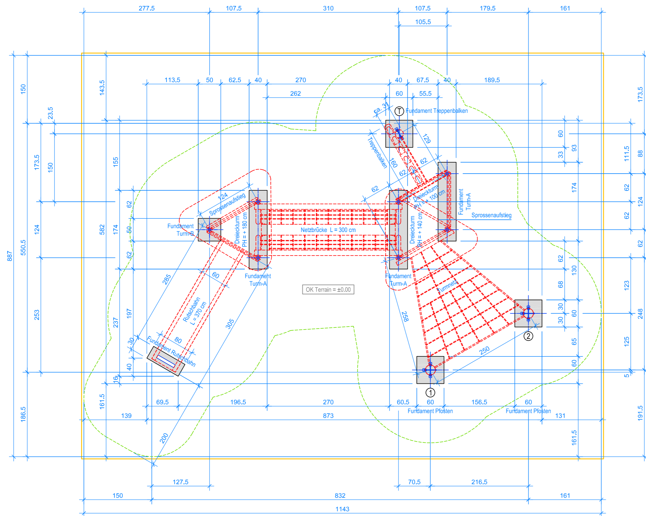
GRUNDRISS 1:50
