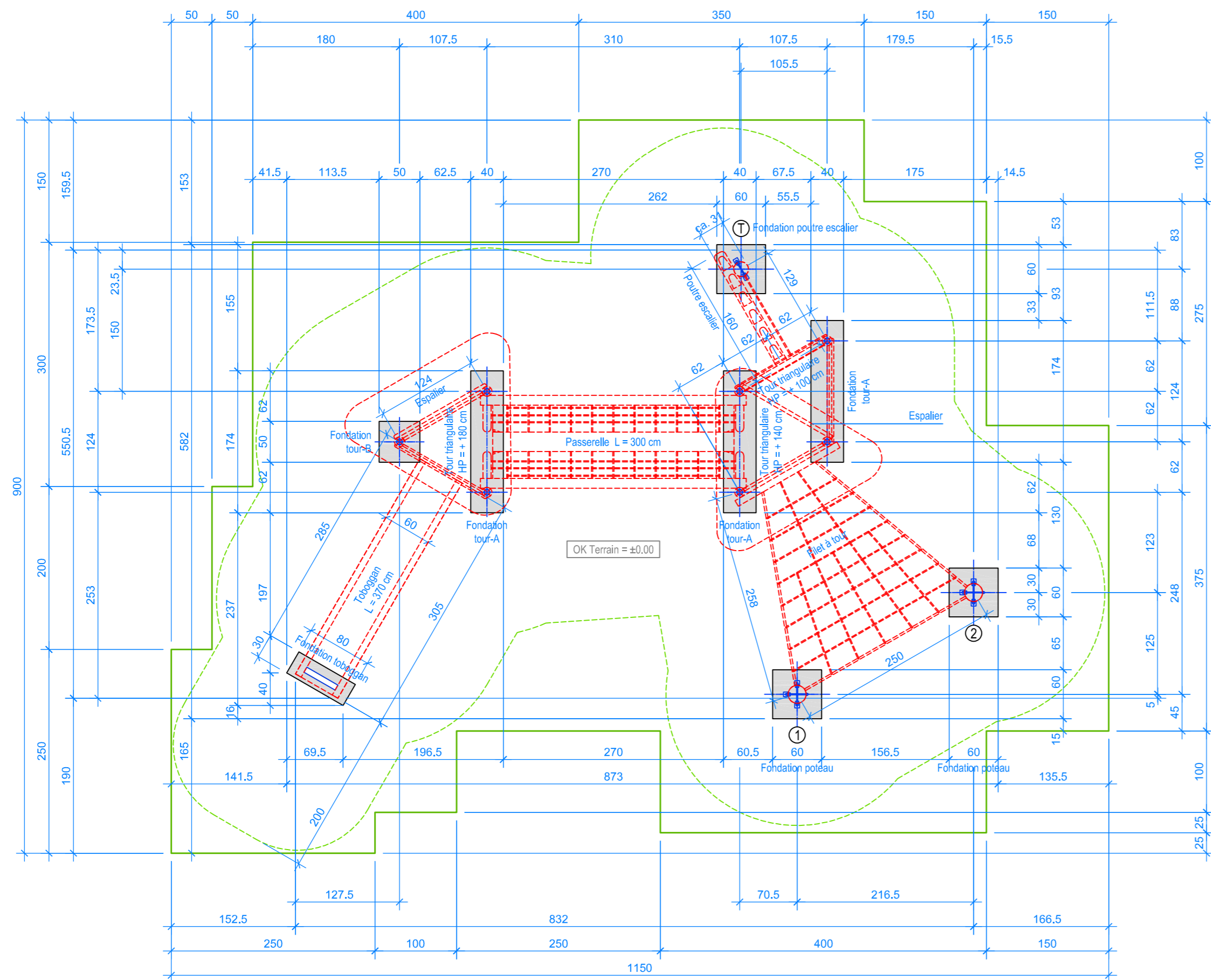
PLAN 1:50
