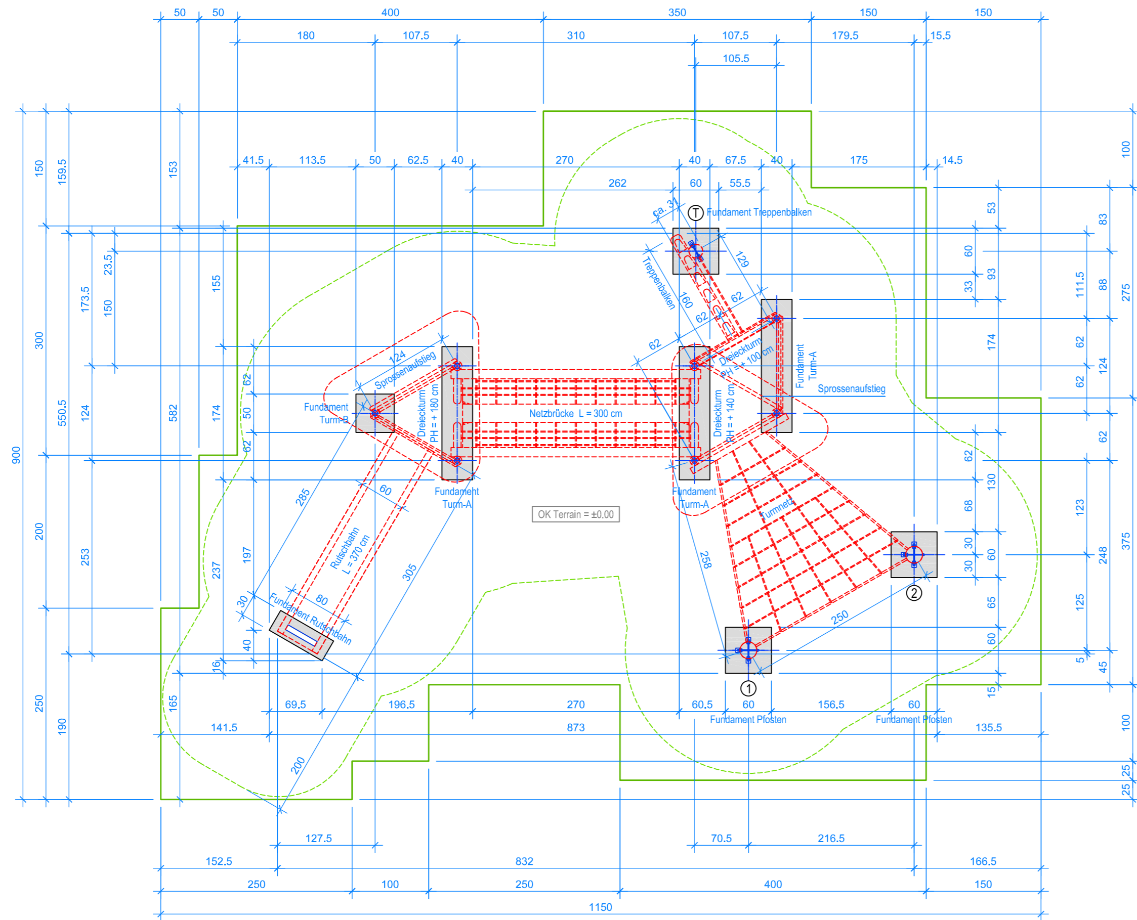
GRUNDRISS 1:50
