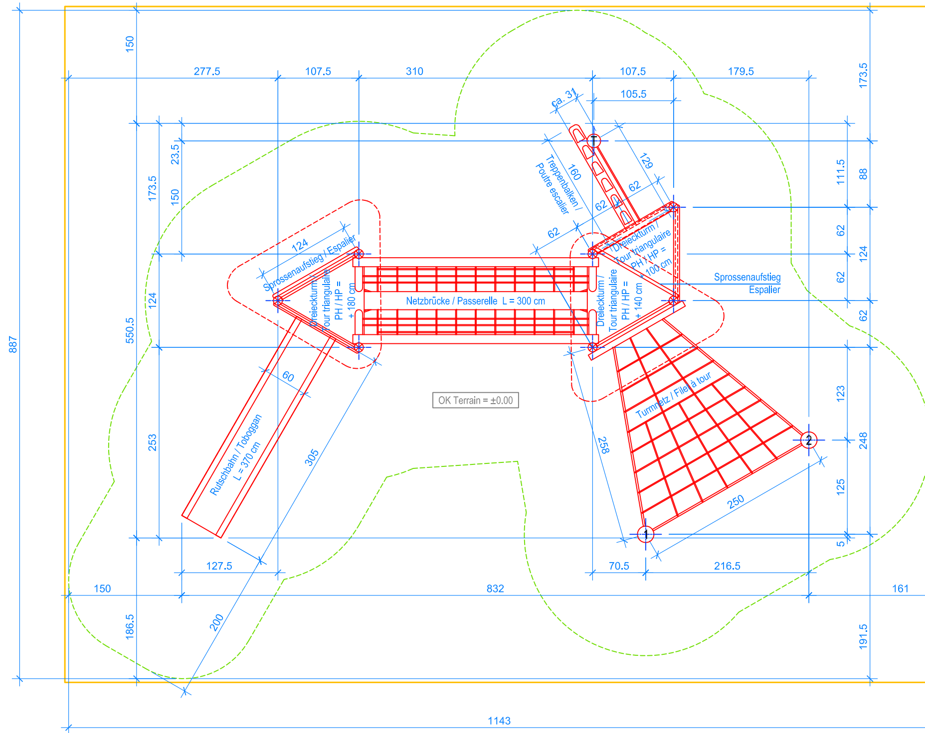
GRUNDRISS / PLAN 1:50
