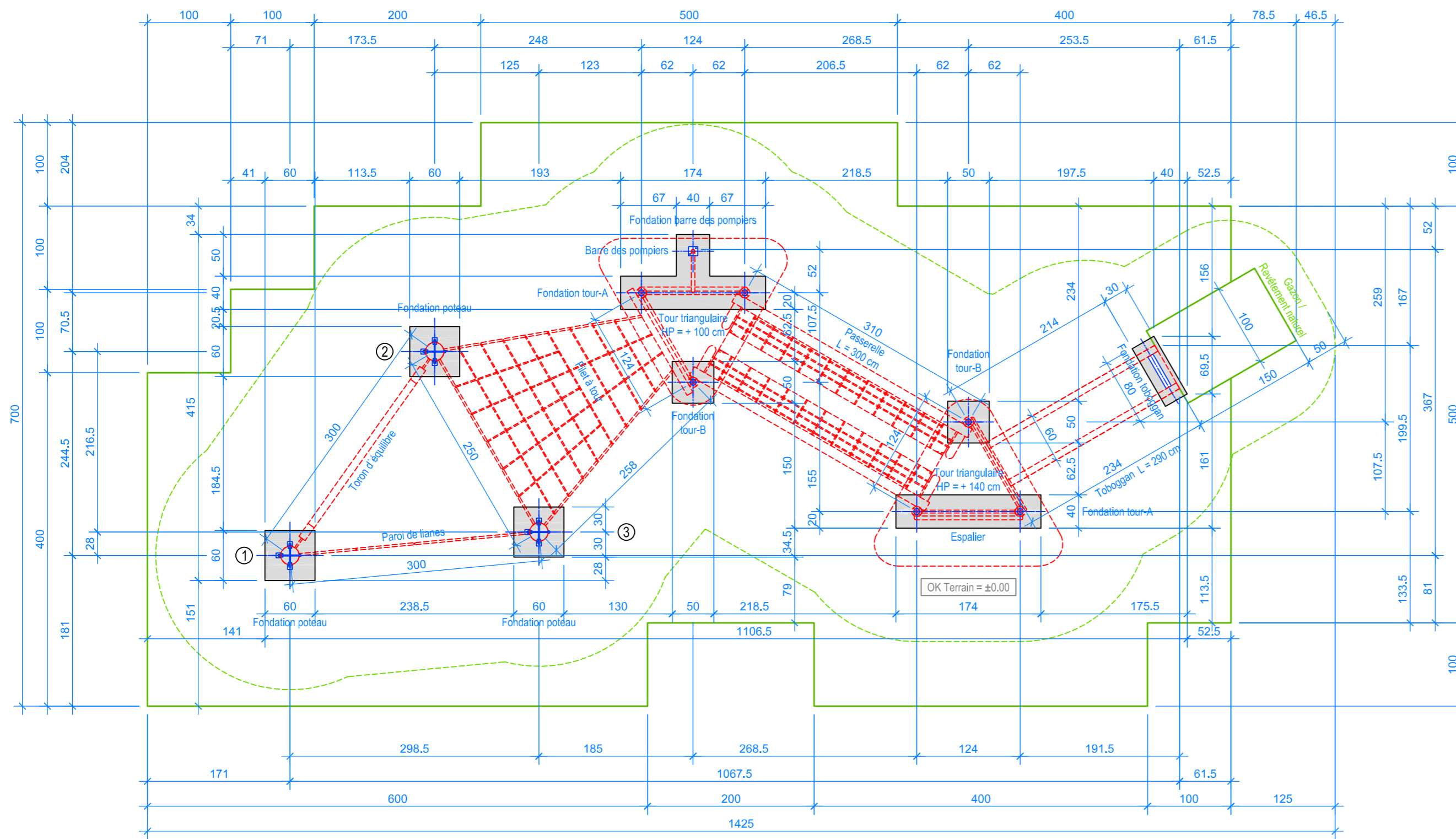
PLAN 1:50
