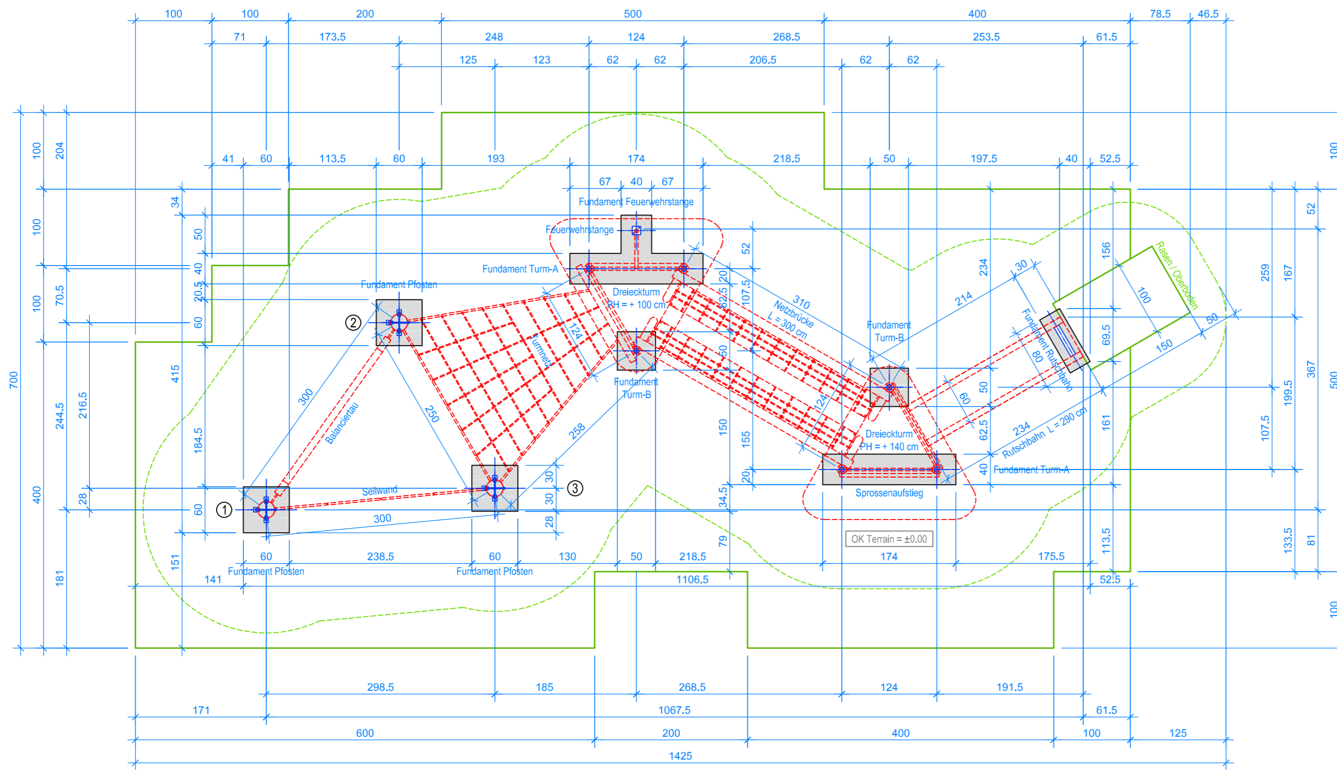
GRUNDRISS 1:50
