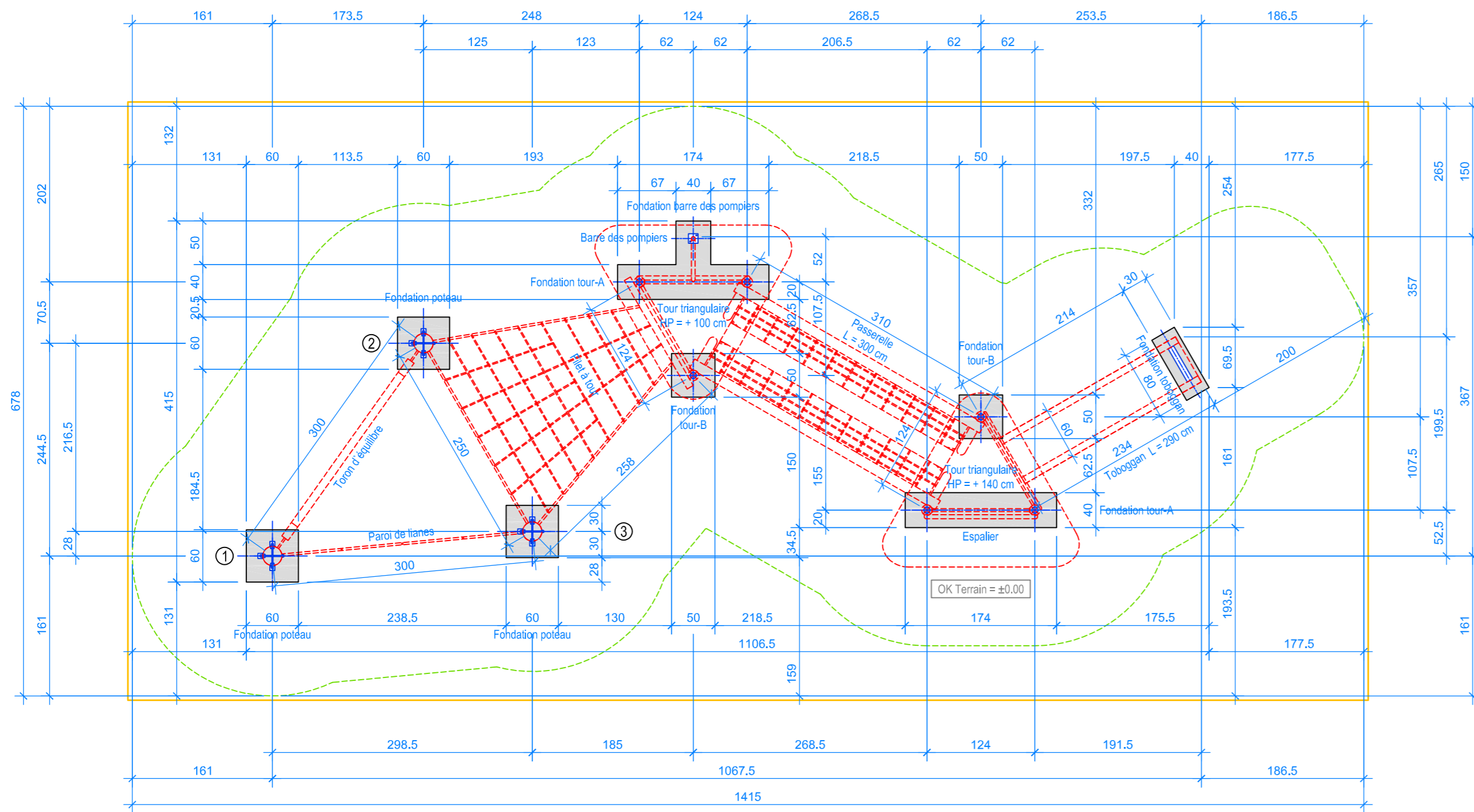
PLAN 1:50
