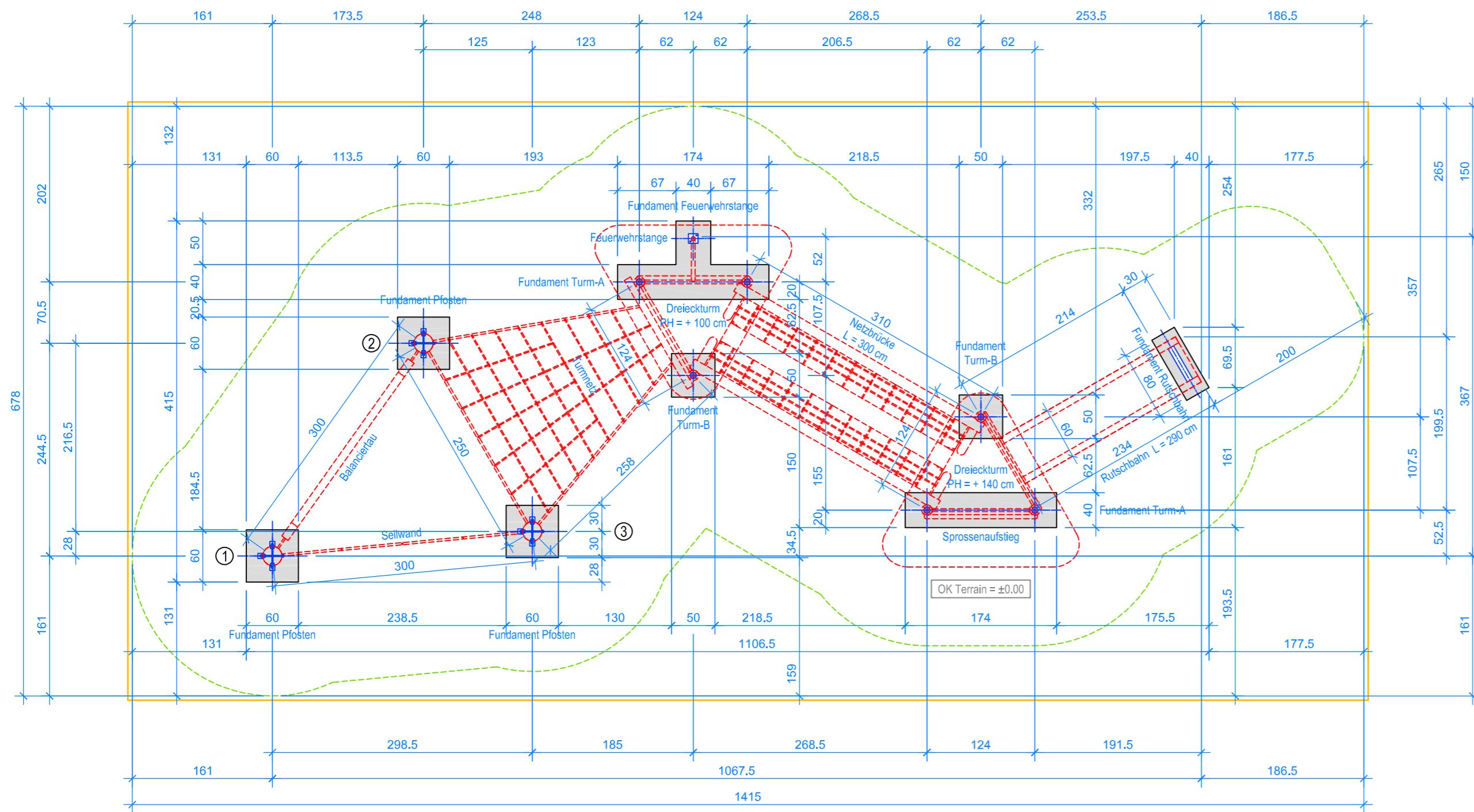
GRUNDRISS 1:50
