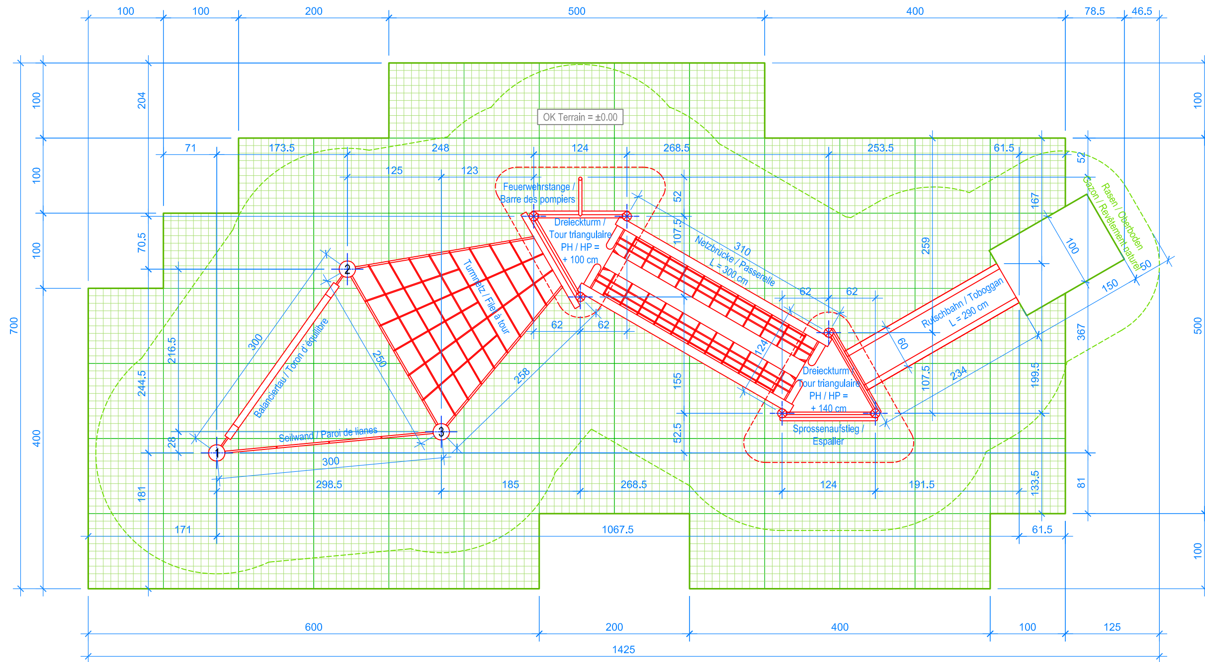
GRUNDRISS / PLAN 1:50
