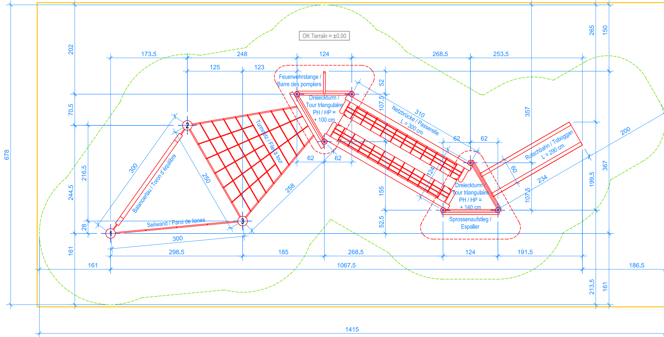
GRUNDRISS / PLAN 1:50
