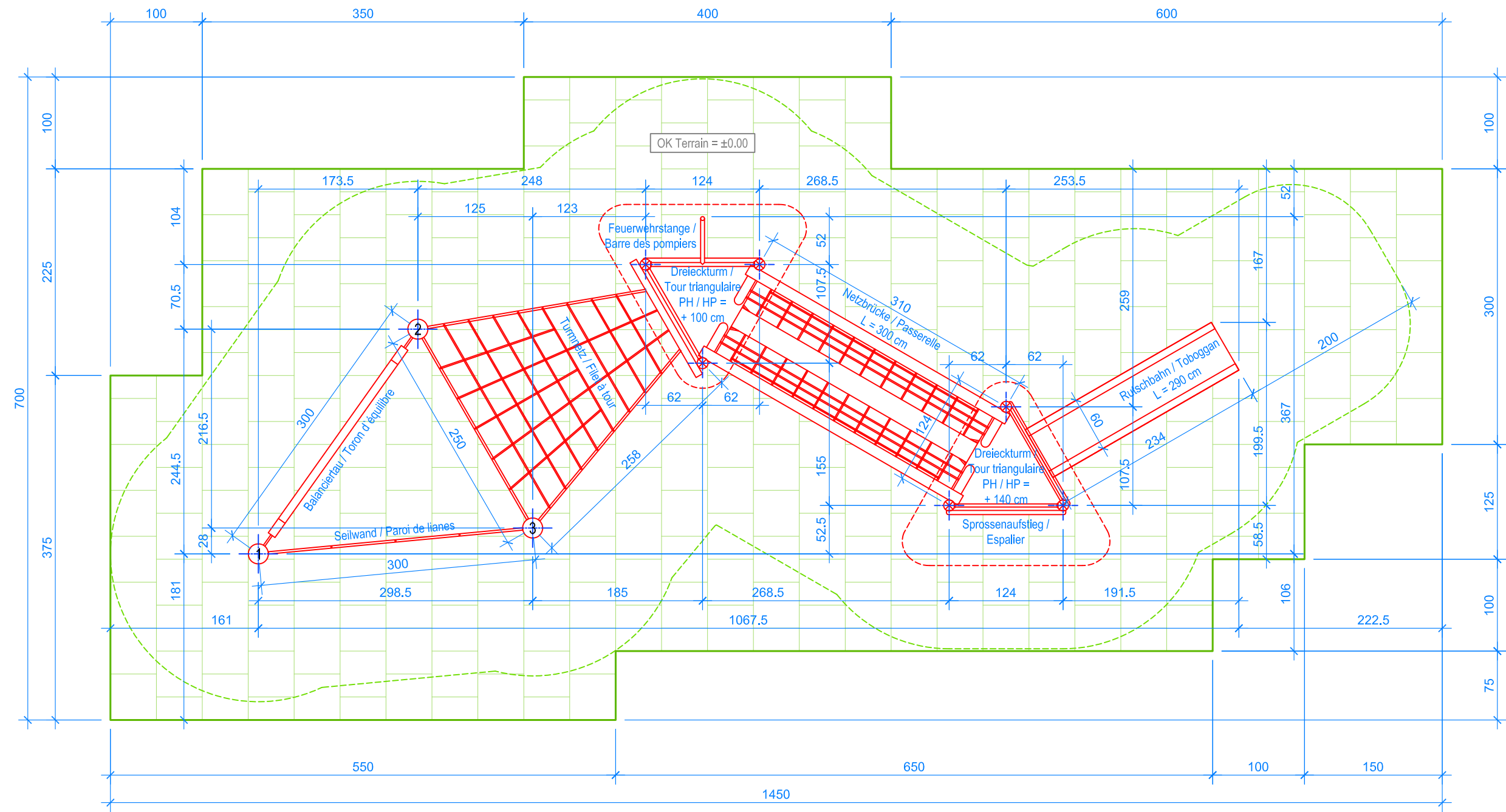
GRUNDRISS / PLAN 1:50
