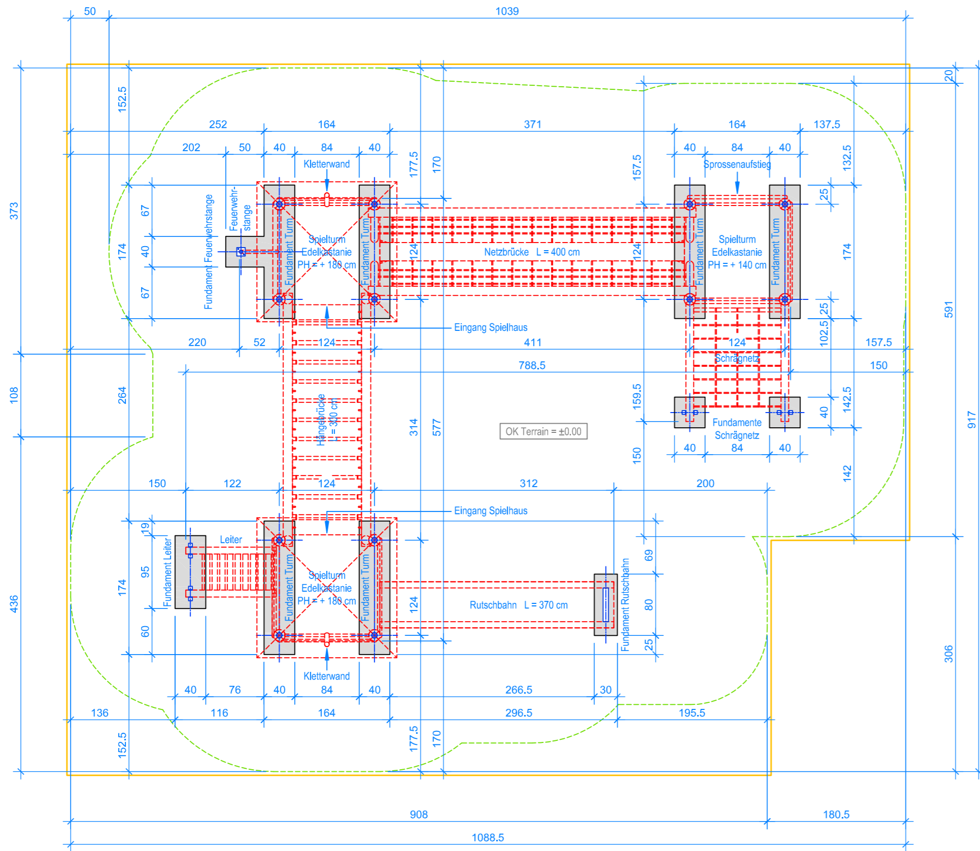
GRUNDRISS 1:50
