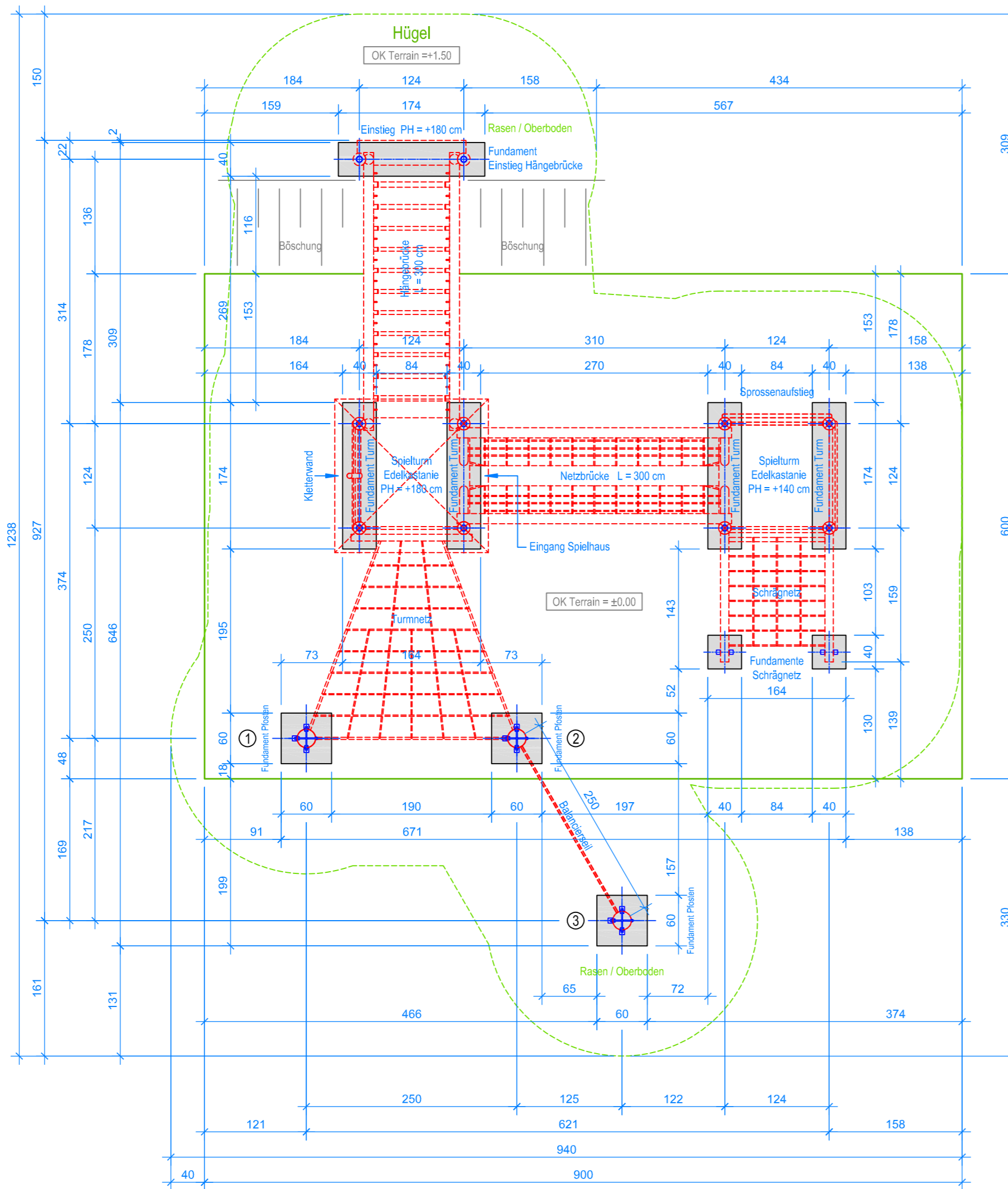
GRUNDRISS 1:50
