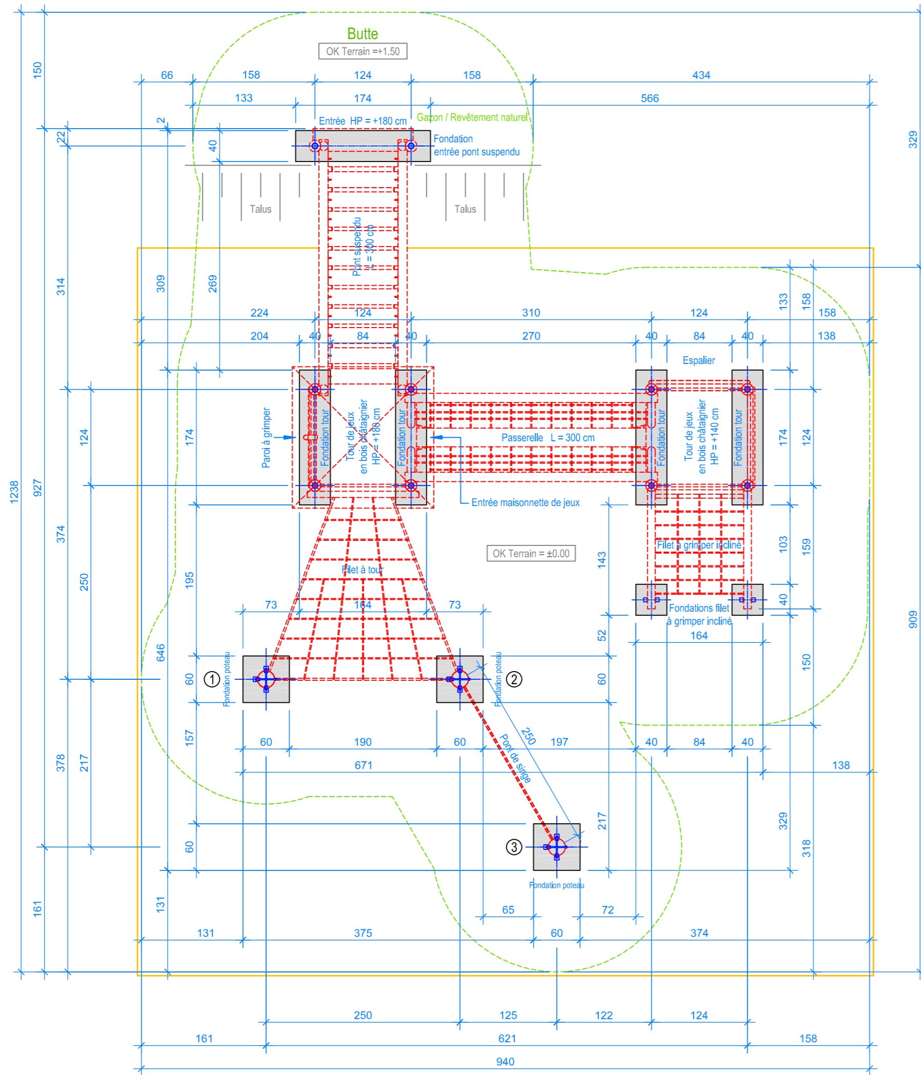
PLAN 1:50
