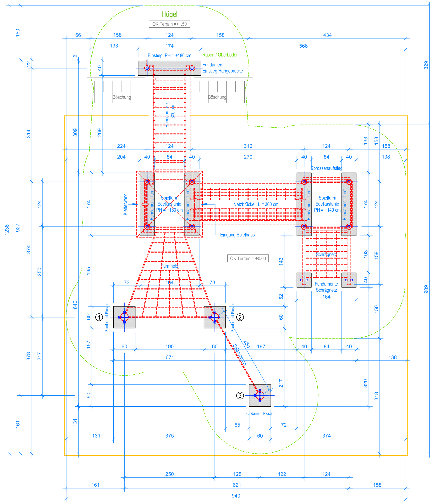
GRUNDRISS 1:50
