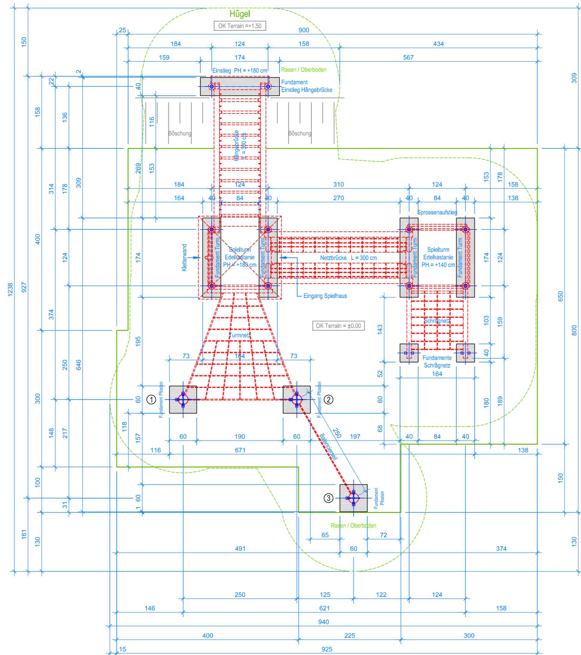
GRUNDRISS 1:50
