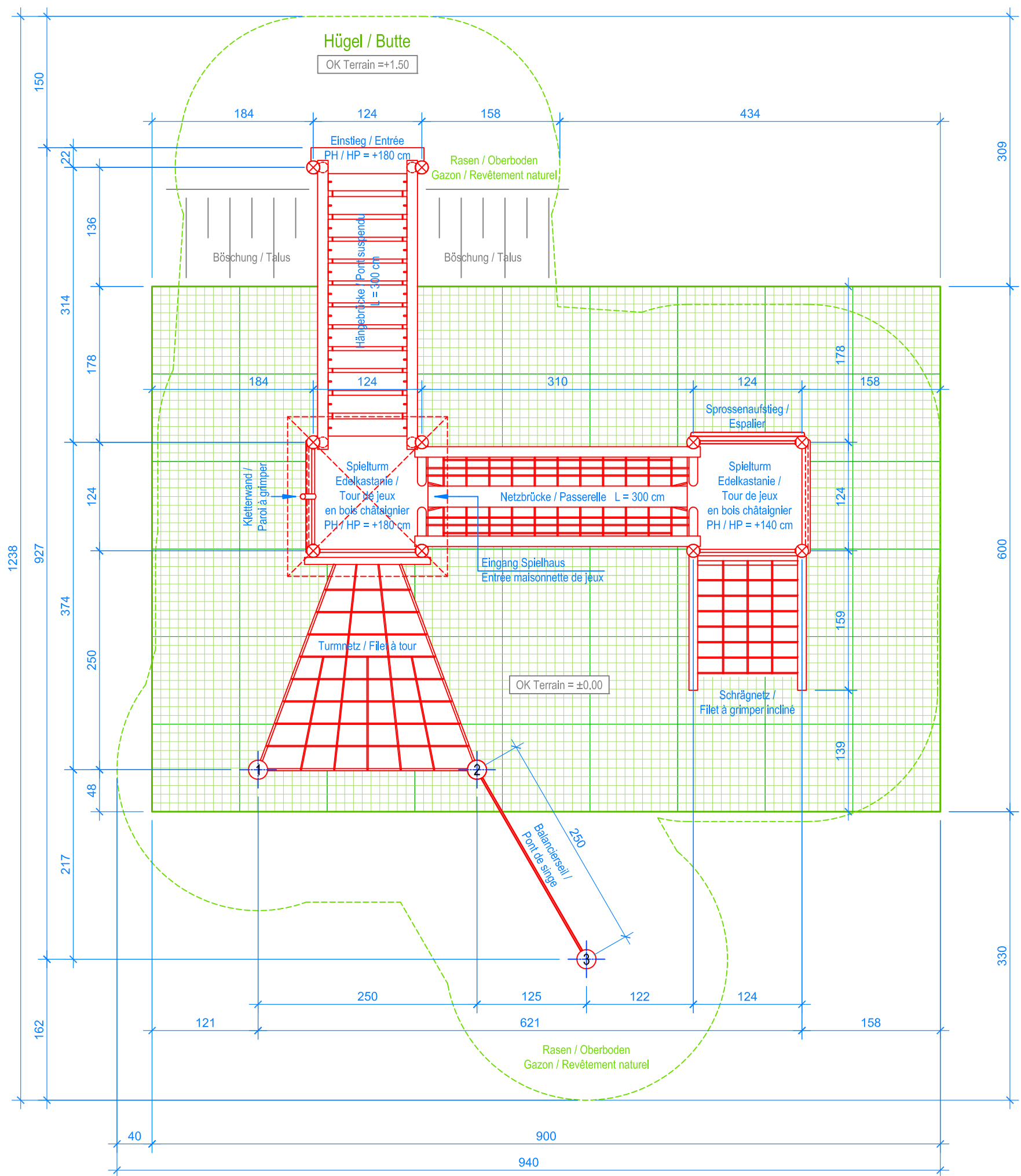
GRUNDRISS / PLAN 1:50
