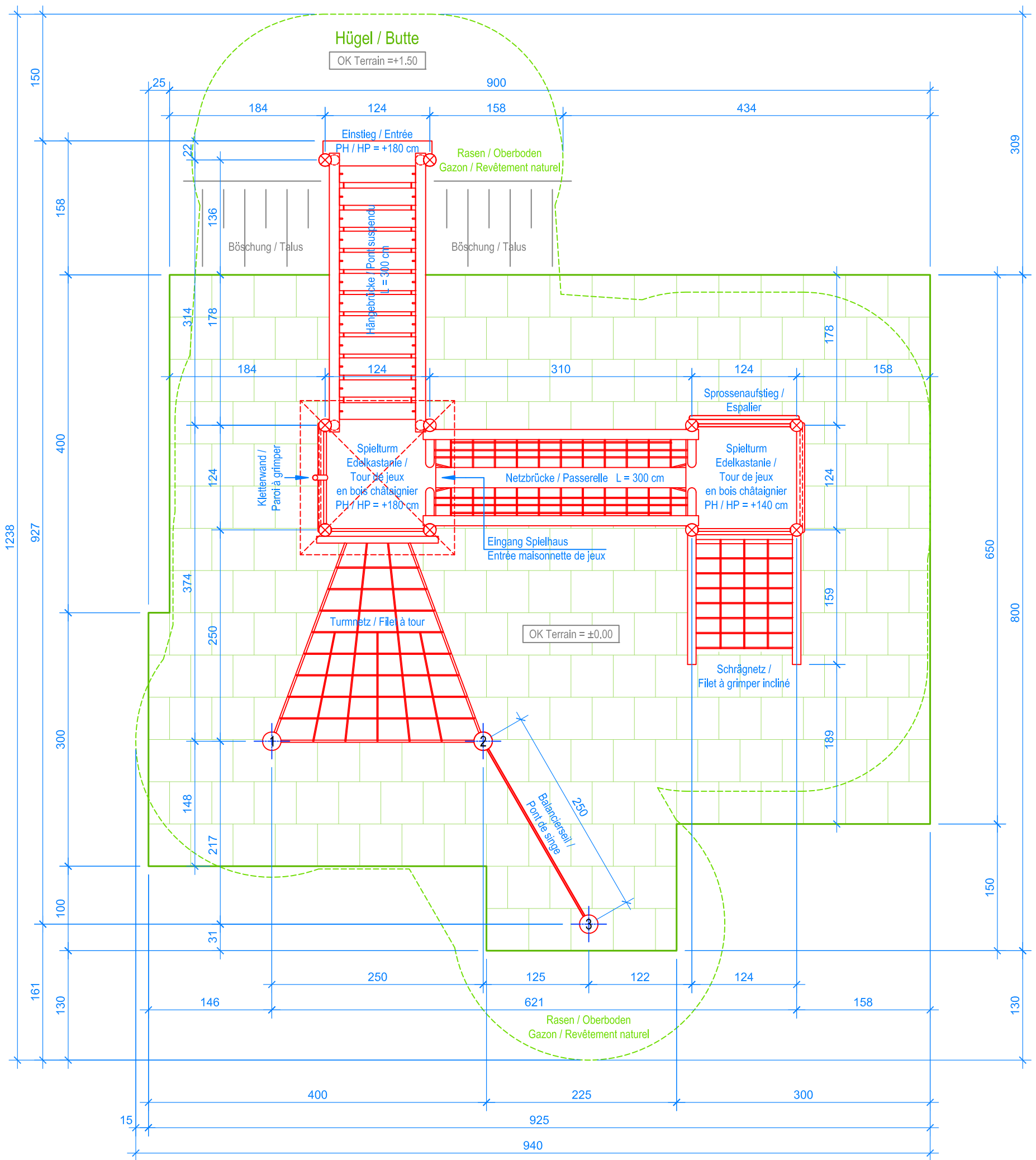
GRUNDRISS / PLAN 1:50
