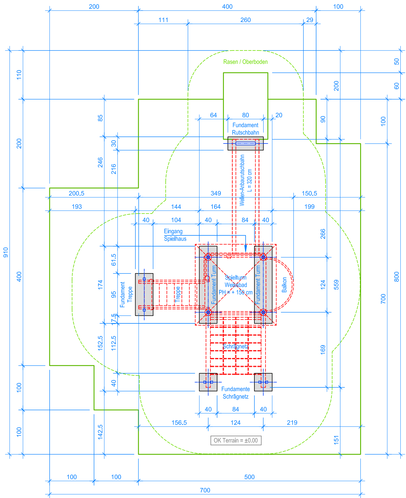
GRUNDRISS 1:50
