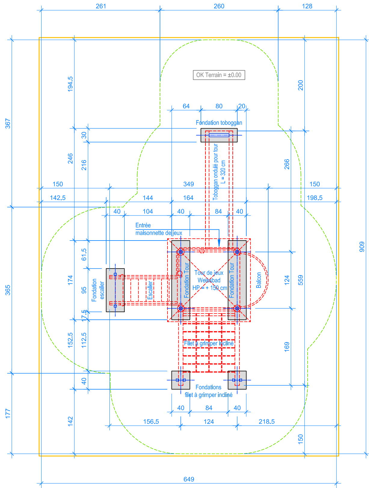
PLAN 1:50
