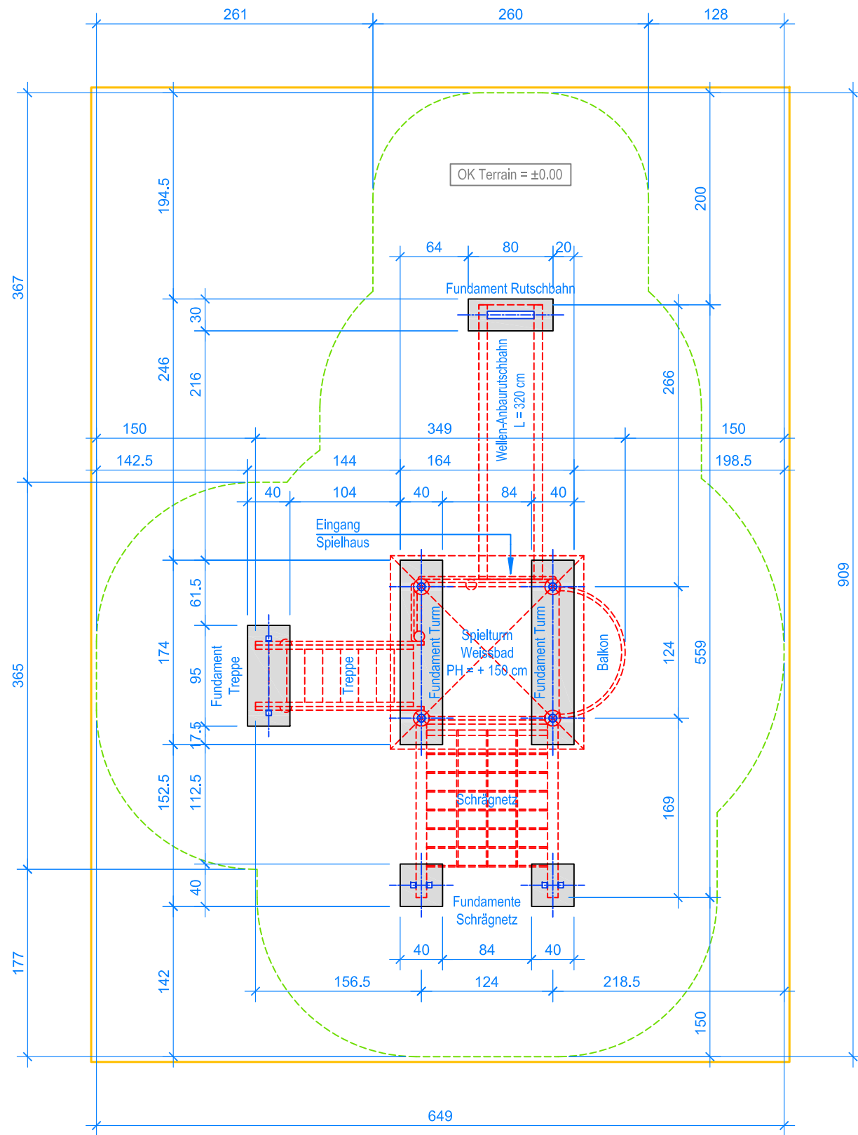
GRUNDRISS 1:50
