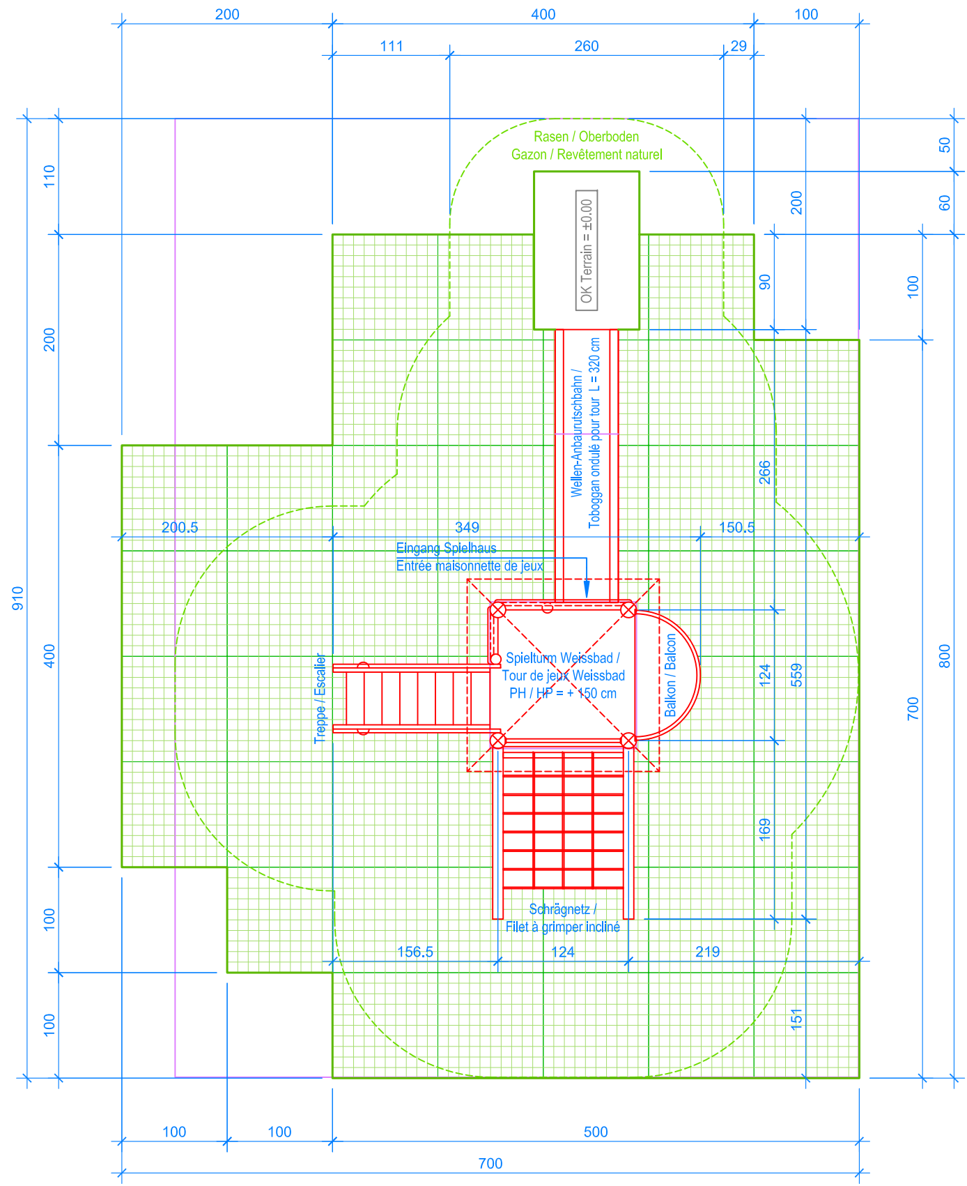
GRUNDRISS / PLAN 1:50
