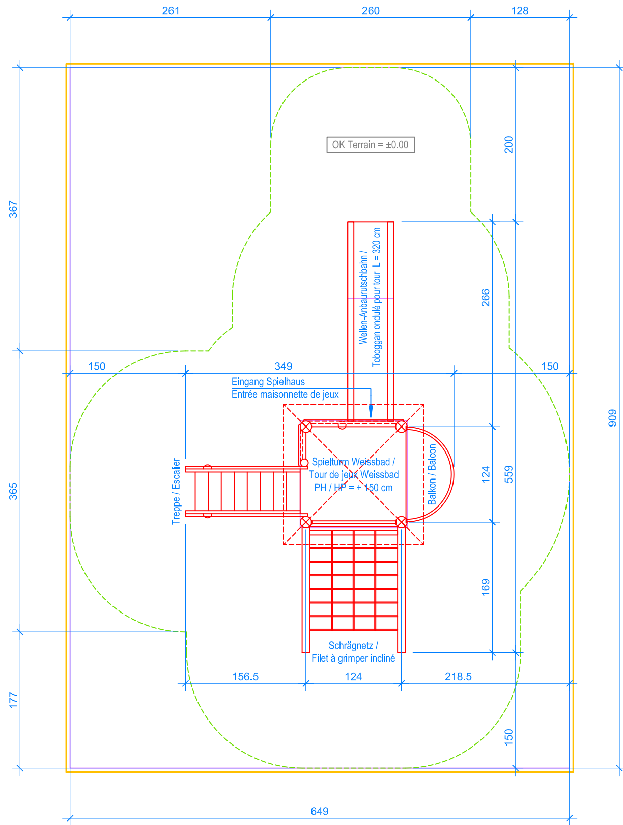
GRUNDRISS / PLAN 1:50
