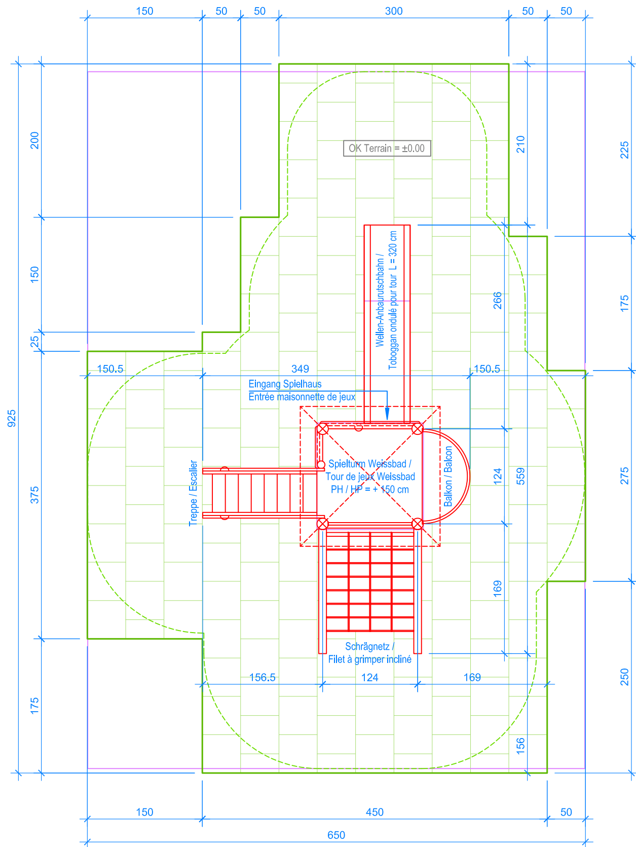
GRUNDRISS / PLAN 1:50
