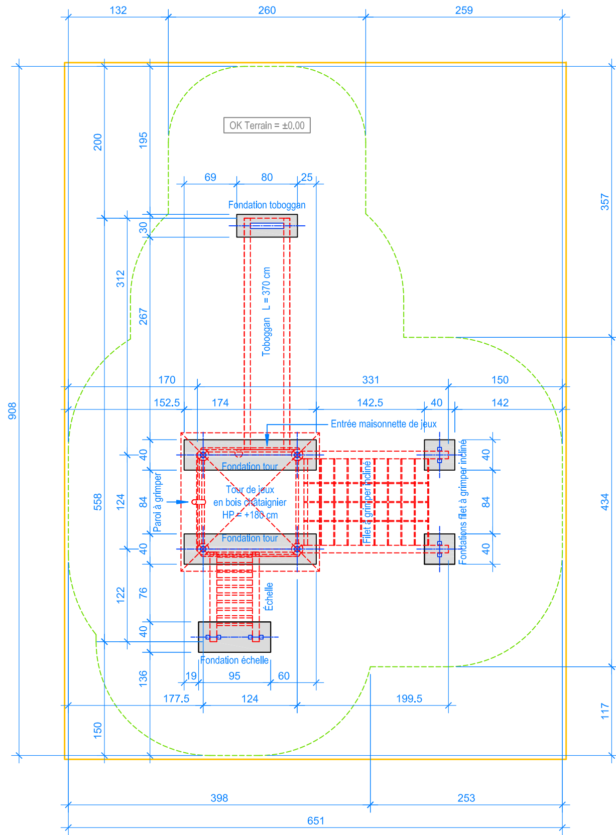
PLAN 1:50
