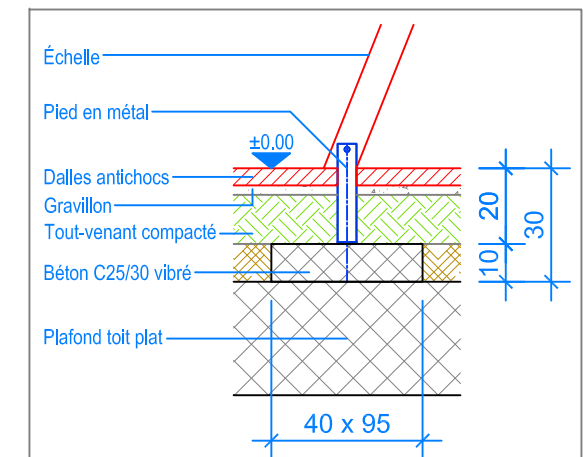
COUPE 1:20 FONDATION ÉCHELLE
