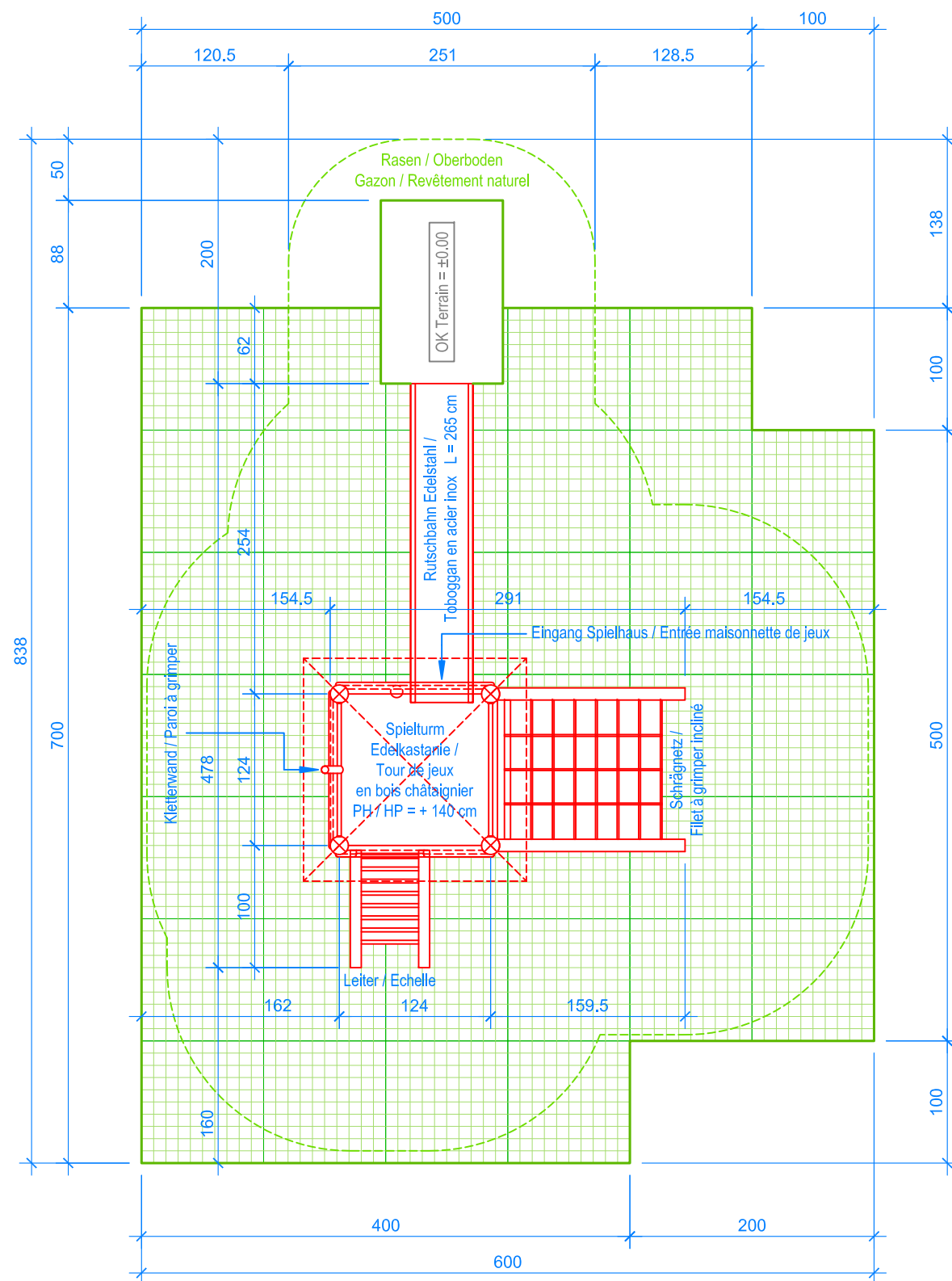
GRUNDRISS / PLAN 1:50
