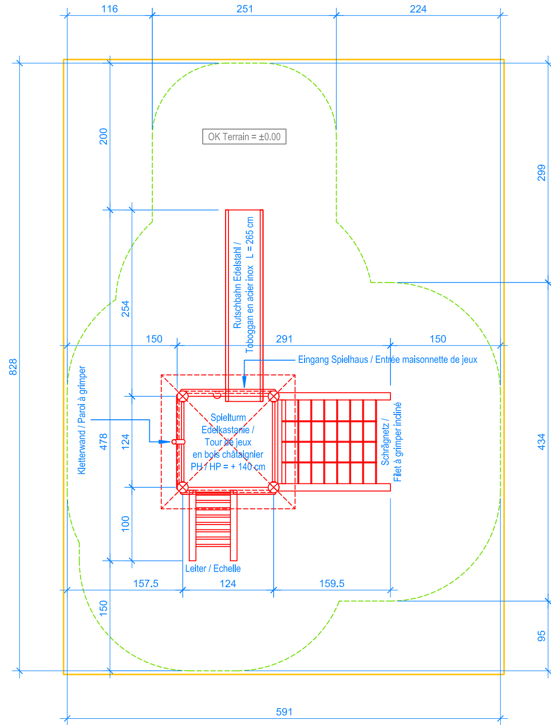
GRUNDRISS / PLAN 1:50
