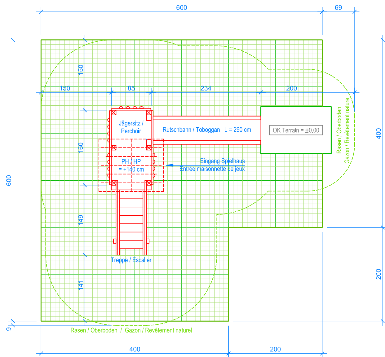
GRUNDRISS / PLAN 1:50
