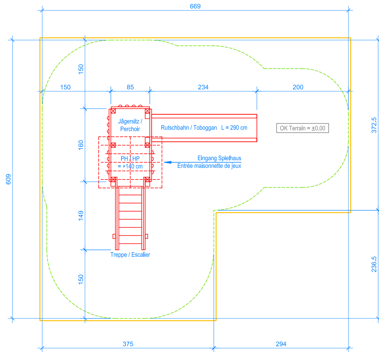
GRUNDRISS / PLAN 1:50
