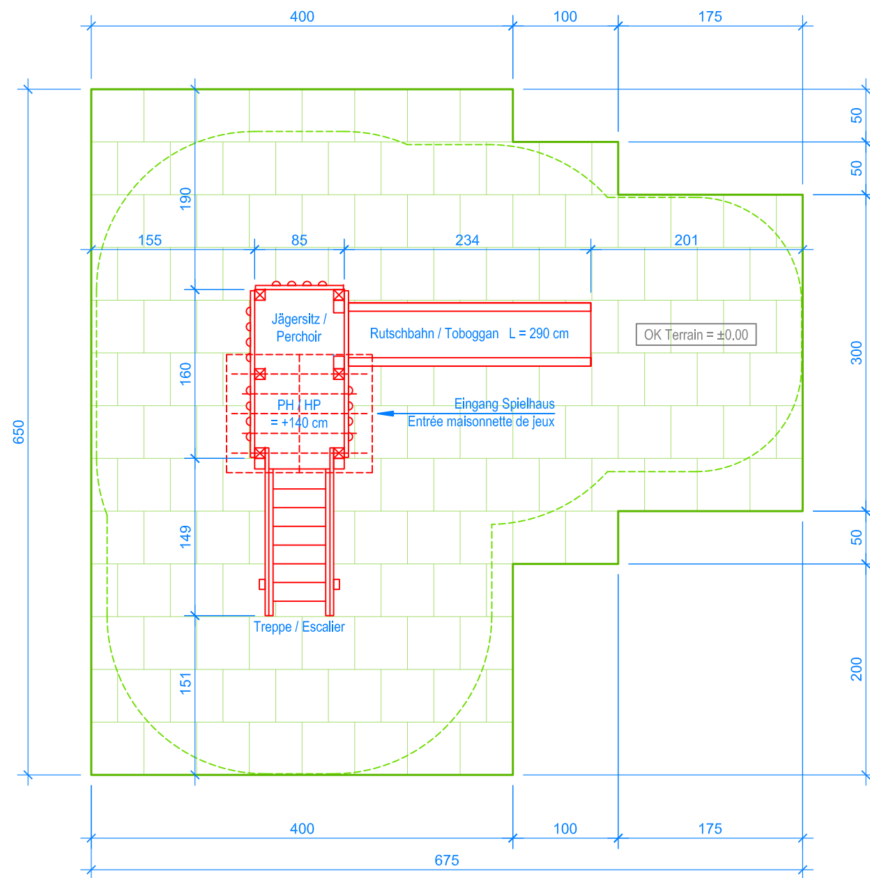
GRUNDRISS / PLAN 1:50
