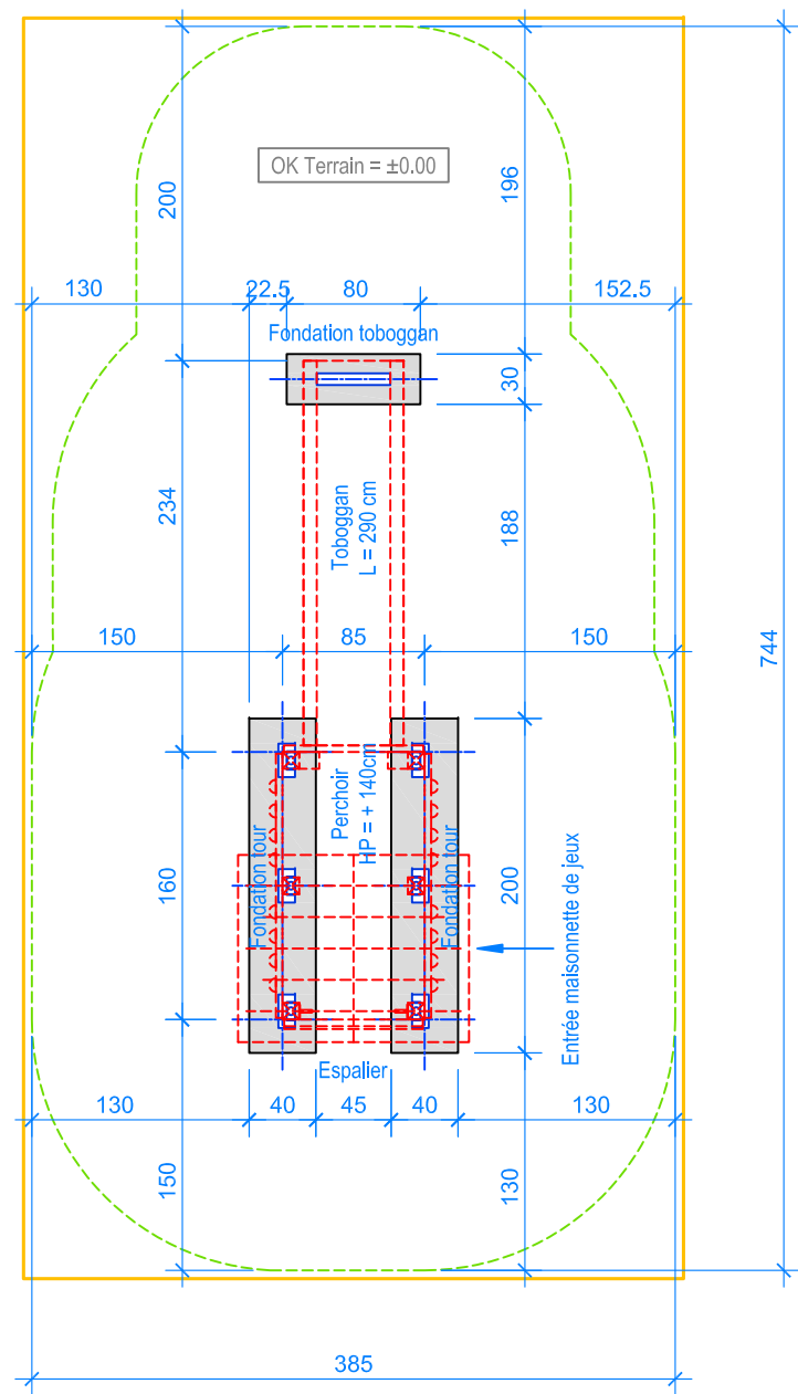
PLAN 1:50
