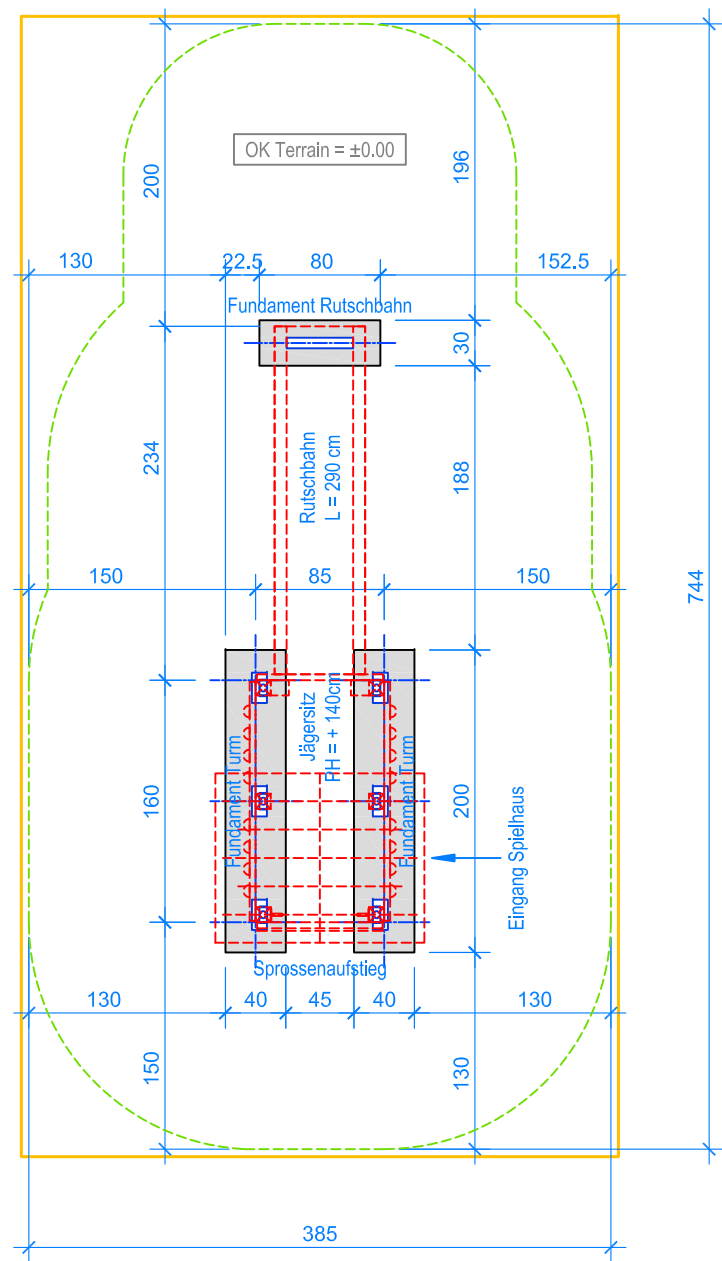
GRUNDRISS 1:50
