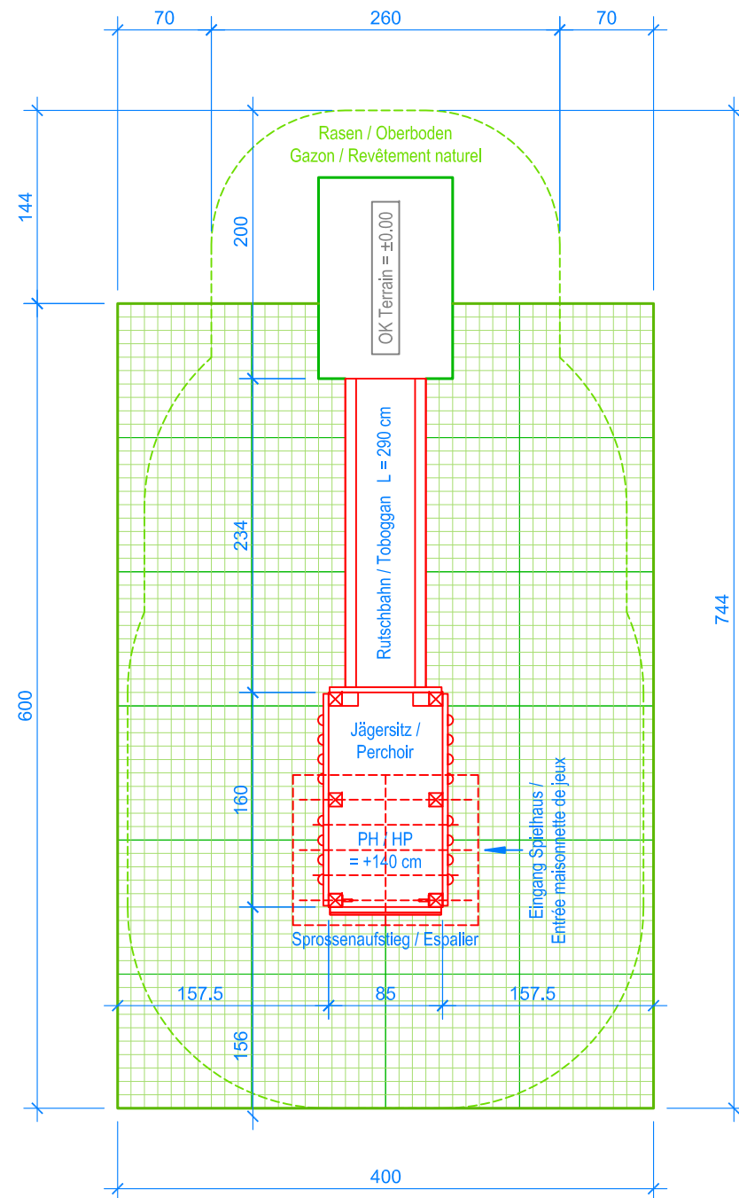
GRUNDRISS / PLAN 1:50
