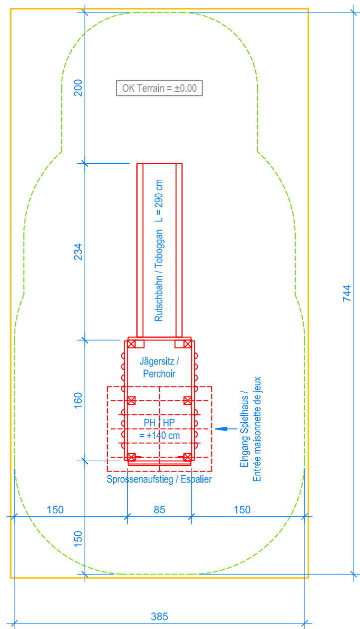
GRUNDRISS / PLAN 1:50
