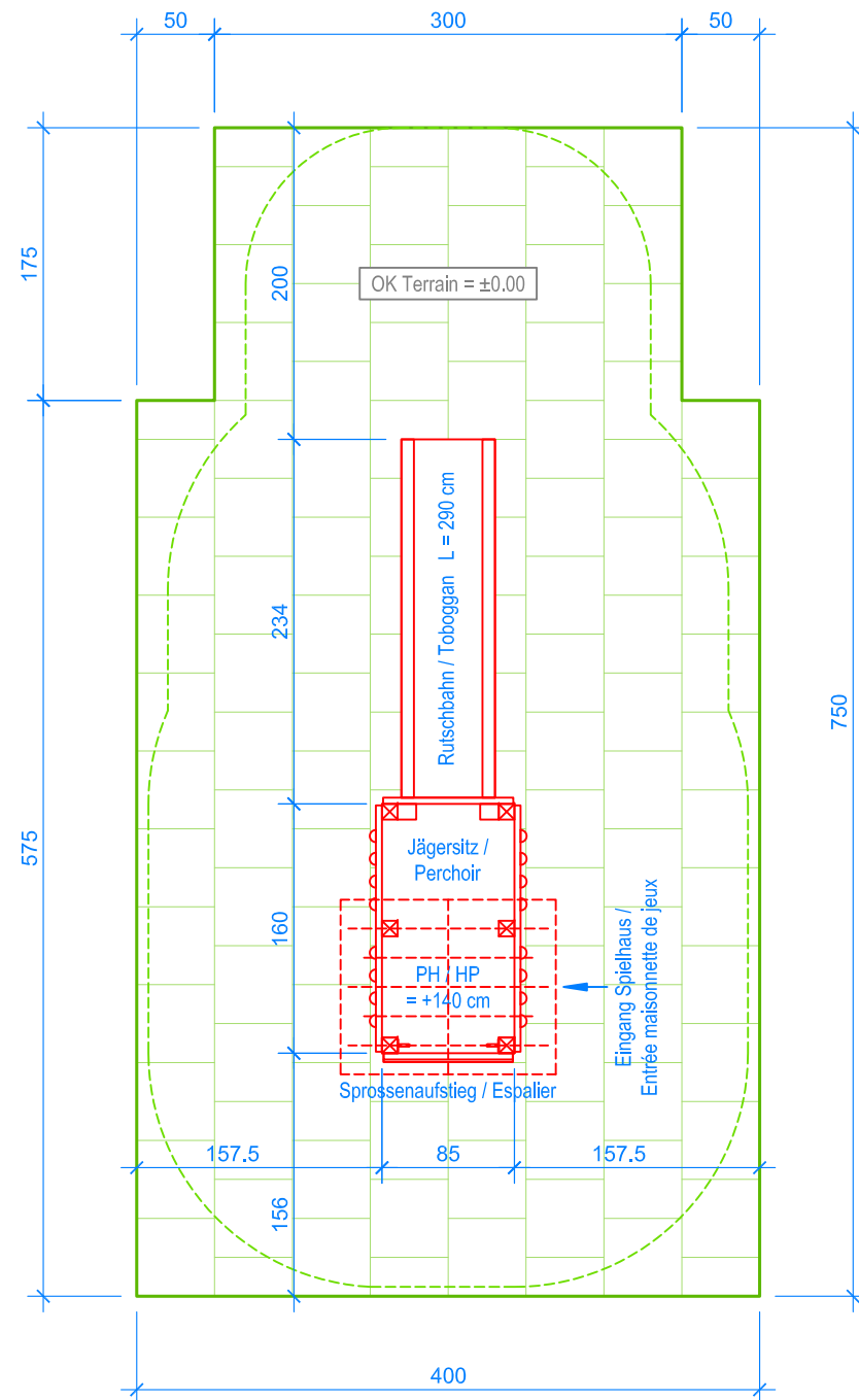
GRUNDRISS / PLAN 1:50
