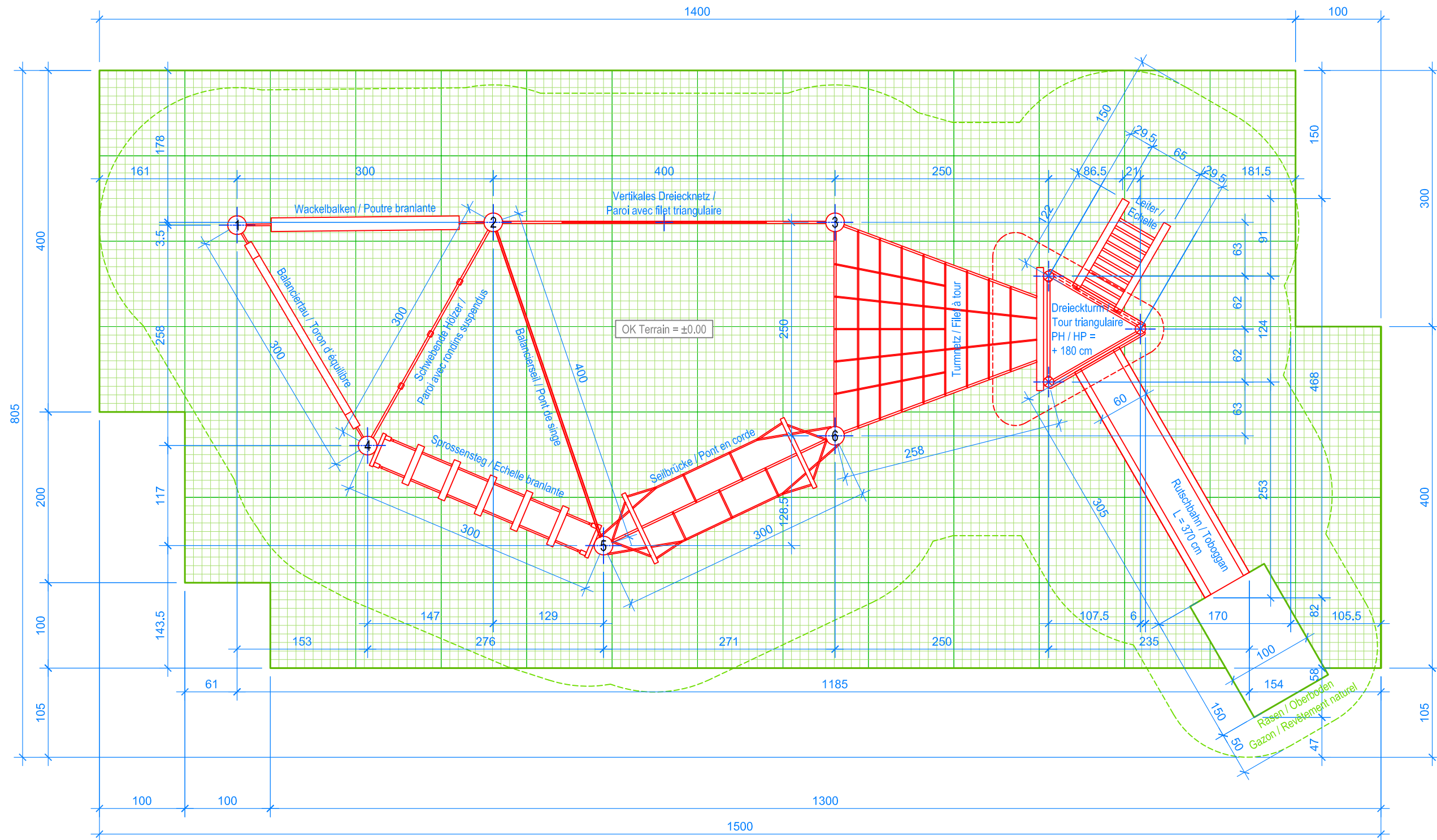
GRUNDRISS / PLAN 1:50
