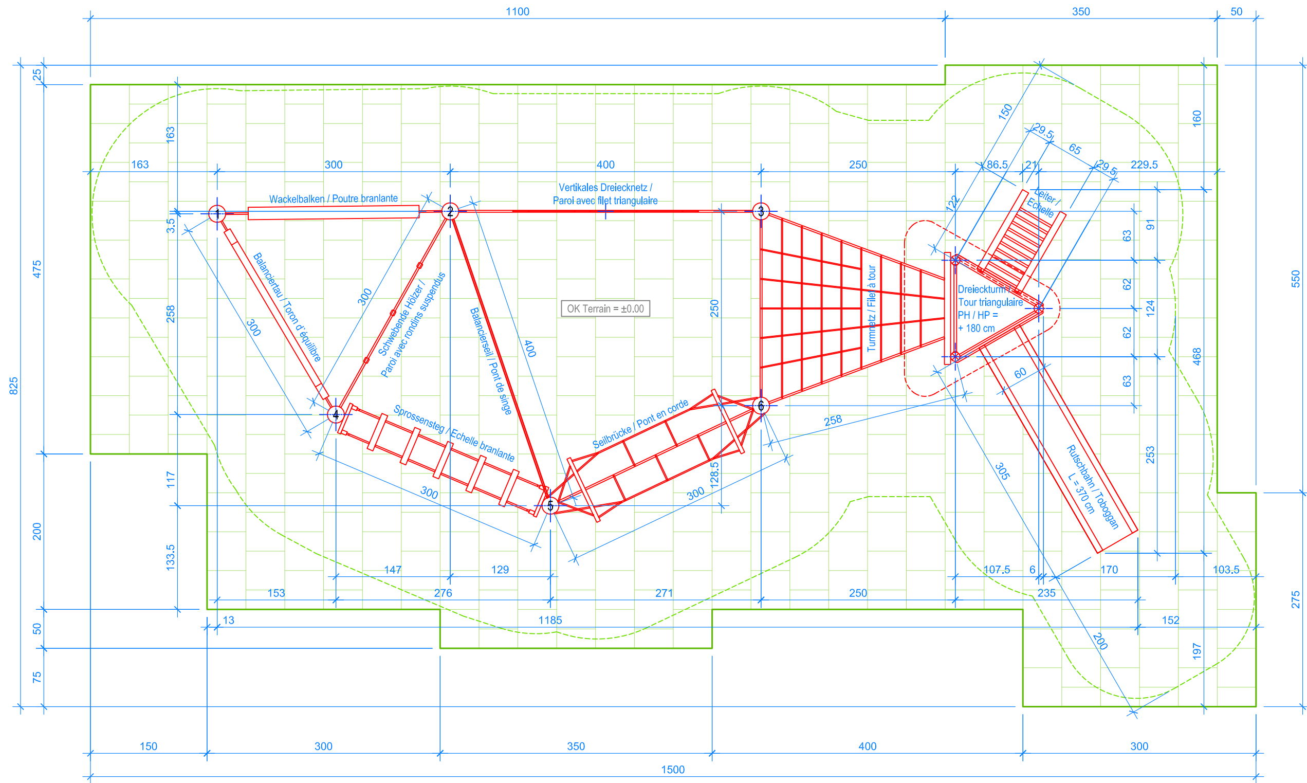
GRUNDRISS / PLAN 1:50
