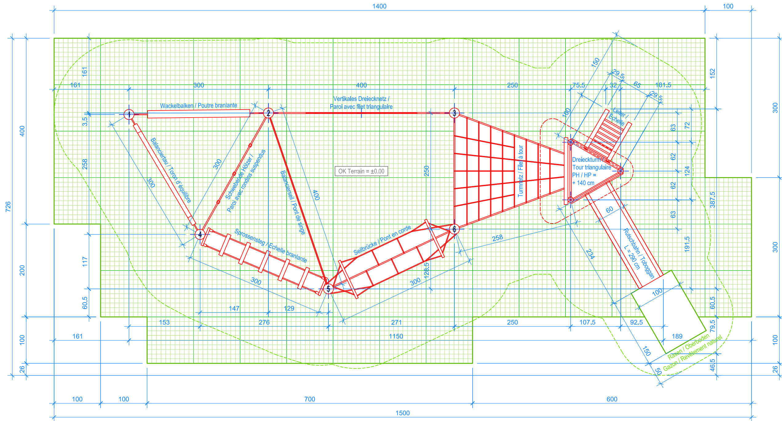
GRUNDRISS / PLAN 1:50
