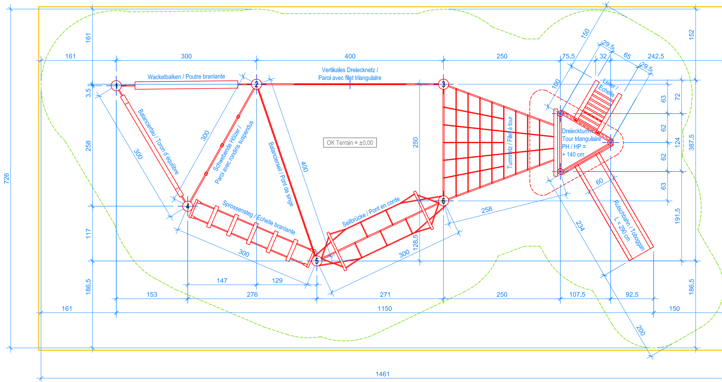
GRUNDRISS / PLAN 1:50
