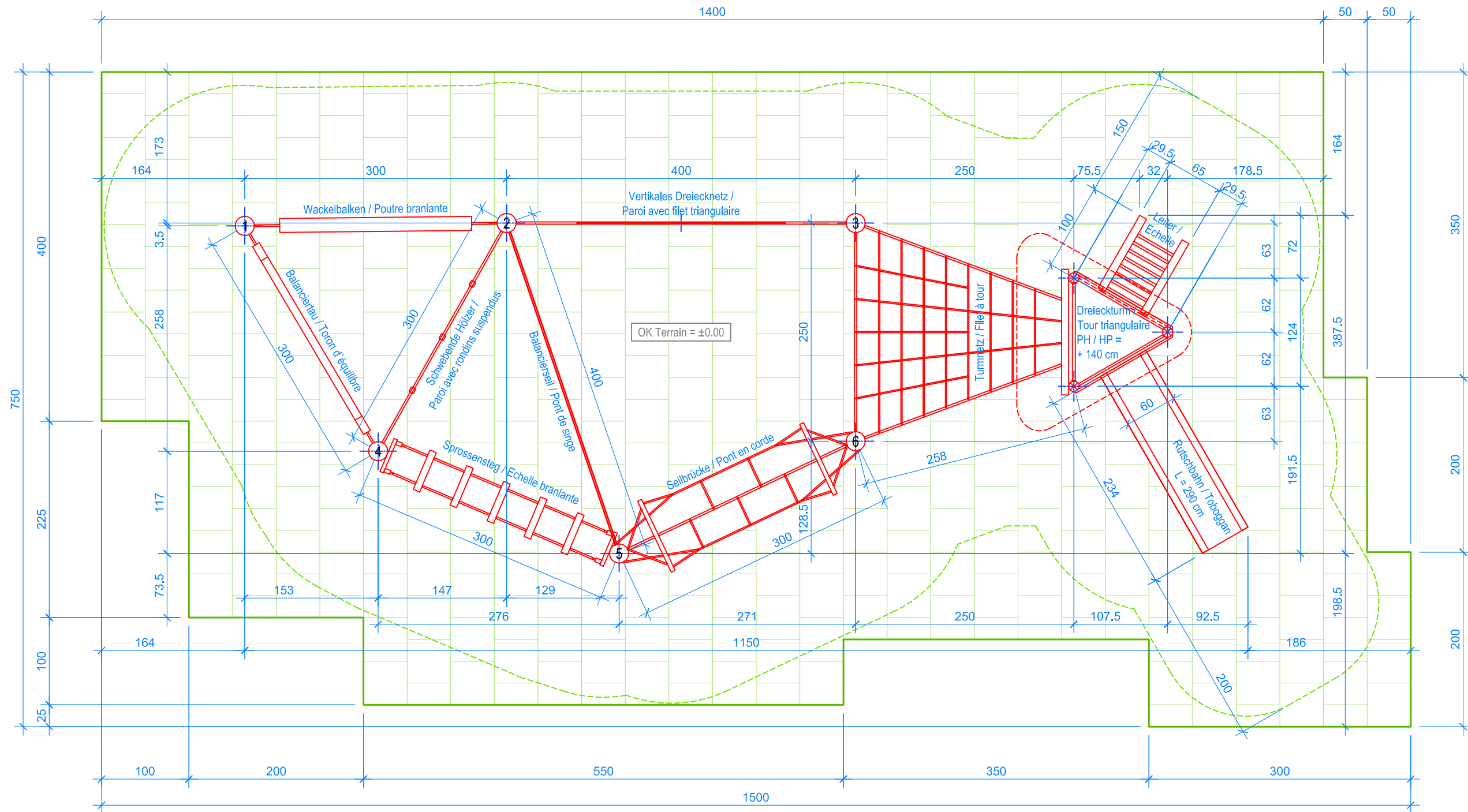
GRUNDRISS / PLAN 1:50
